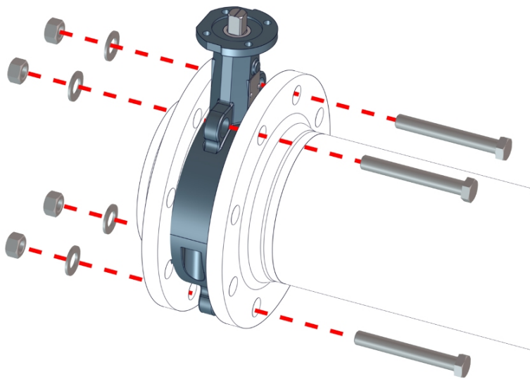
Σχ. 8: Zwischenflanschklappe positionieren
