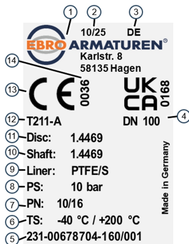
Σχ. 1: Παράδειγμα πινακίδας τύπου
