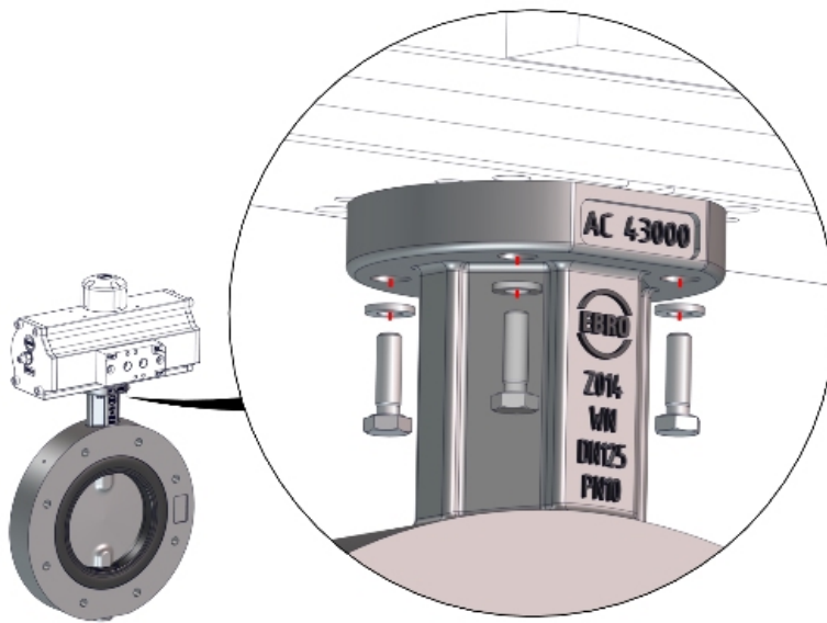
Σχ. 7: Αρχή συναρμολόγησης εξαρτημάτων
