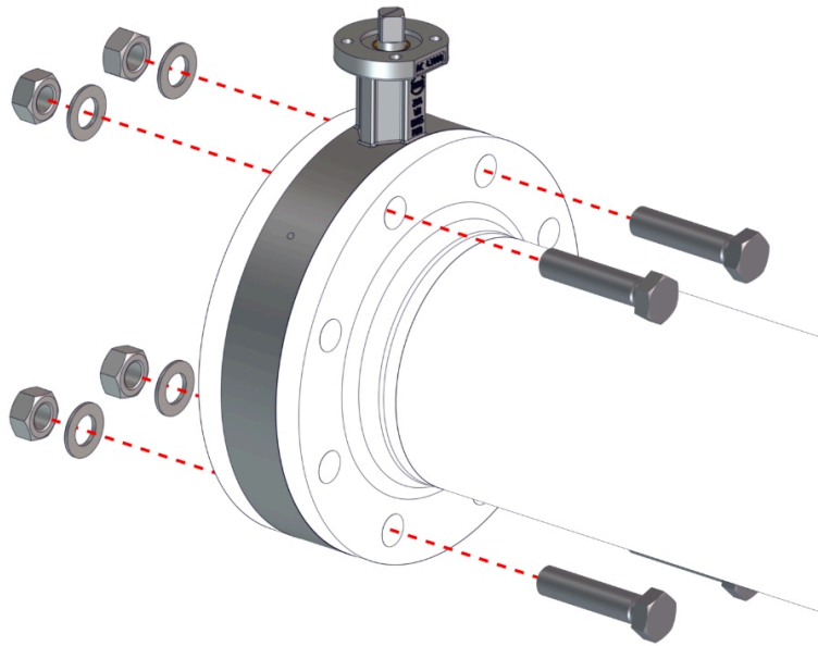
Σχ. 8: Τοποθέτηση βαλβίδας πεταλούδας τύπου full lug
