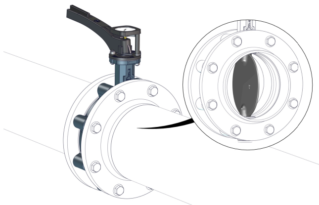
Σχ. 13: Έκπλυση σωλήνα
