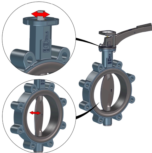
Σχ. 4: Κινούμενα μέρη
