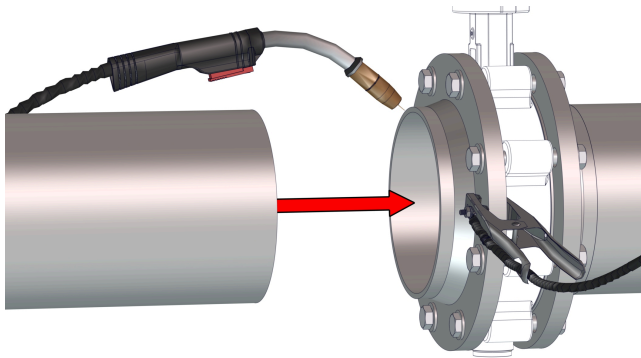
Σχ. 10: Συγκολλήστε τον σωλήνα με τη φλάντζα
