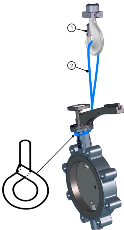
Σχ. 6: Ανύψωση βαλβίδας πεταλούδας τύπου lug
