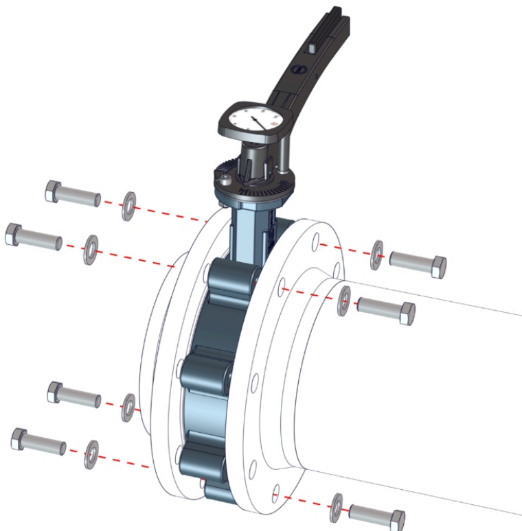
Σχ. 8: Τοποθέτηση βαλβίδας πεταλούδας τύπου lug
