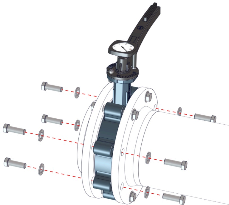
Σχ. 9: Βιδώστε τη βαλβίδα πεταλούδας τύπου lug
