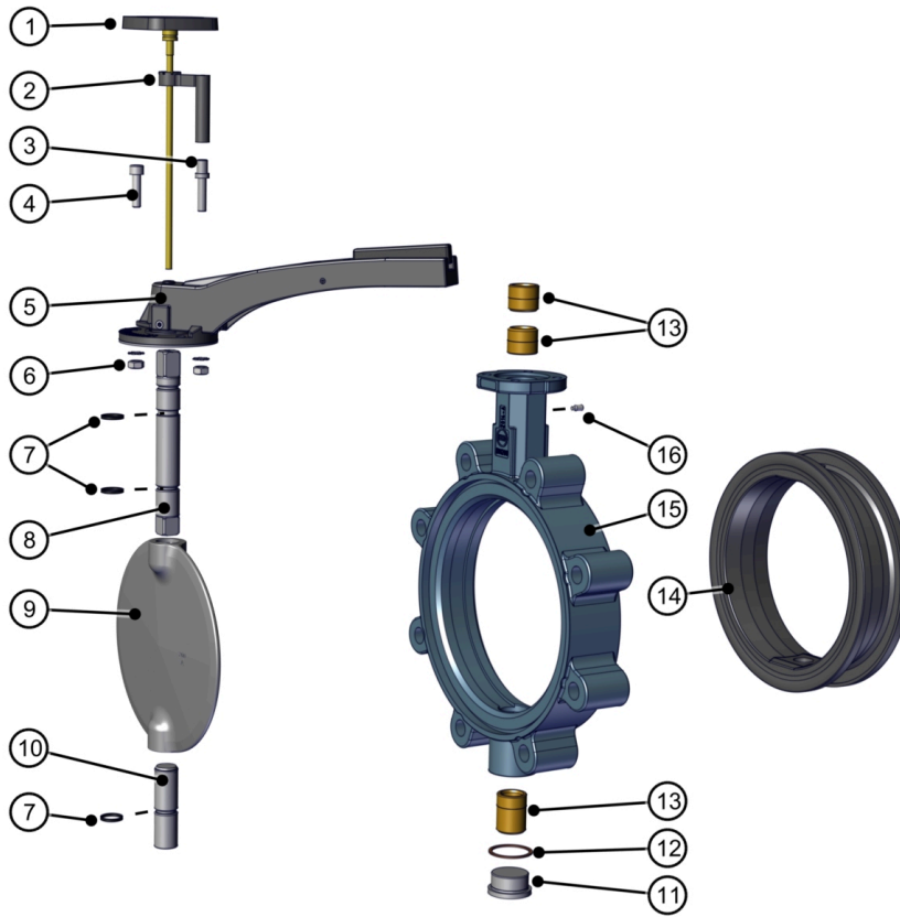
Σχ. 16: Λίστα ανταλλακτικών Z014-A THERM
