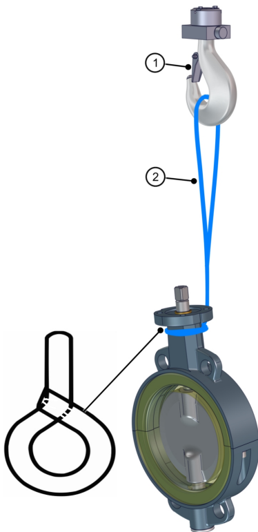
Σχ. 6: Ανύψωση βαλβίδας πεταλούδας τύπου wafer
