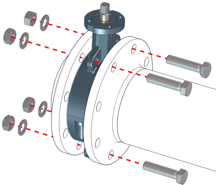
Σχ. 8: Τοποθέτηση βαλβίδας πεταλούδας τύπου wafer
