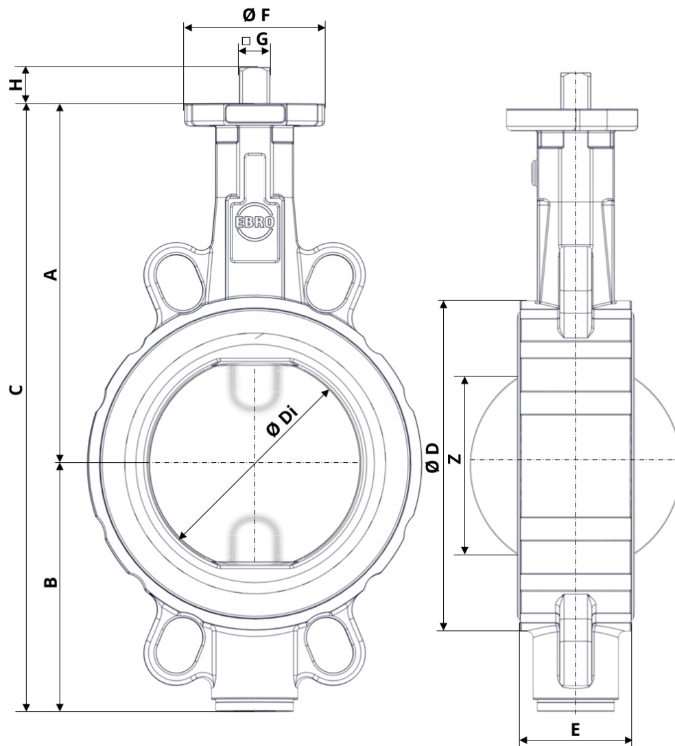
Σχ. 3: Κύριες διαστάσεις Z011-B
