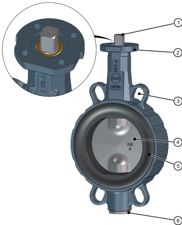
Σχ. 2: Εξαρτήματα
