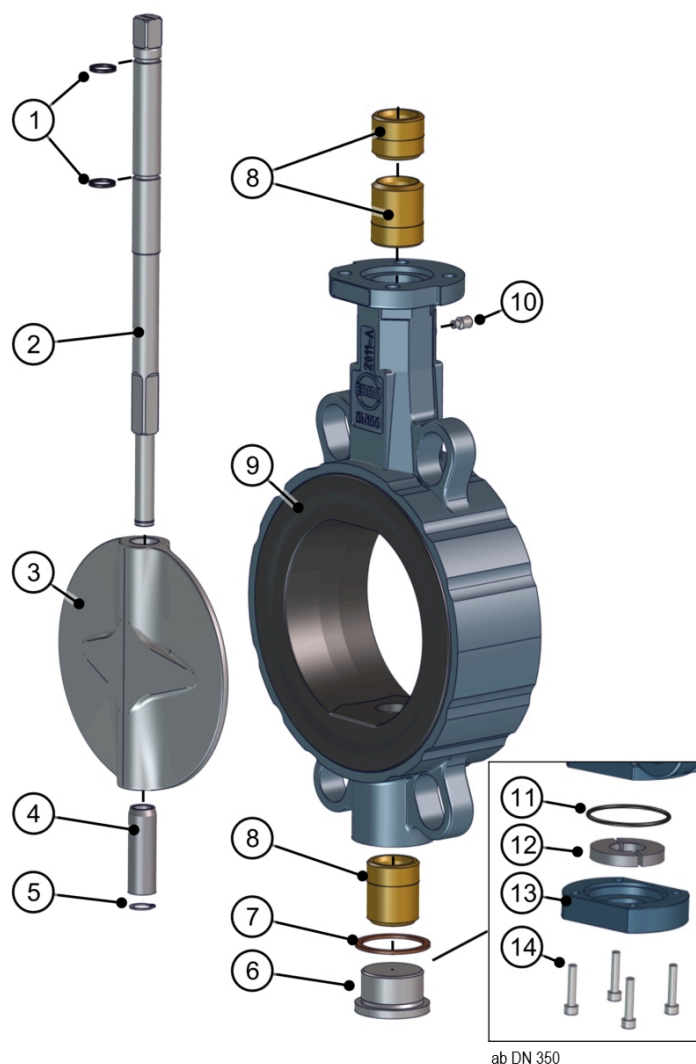
Σχ. 16: Λίστα ανταλλακτικών Z011-B άξονα TS
