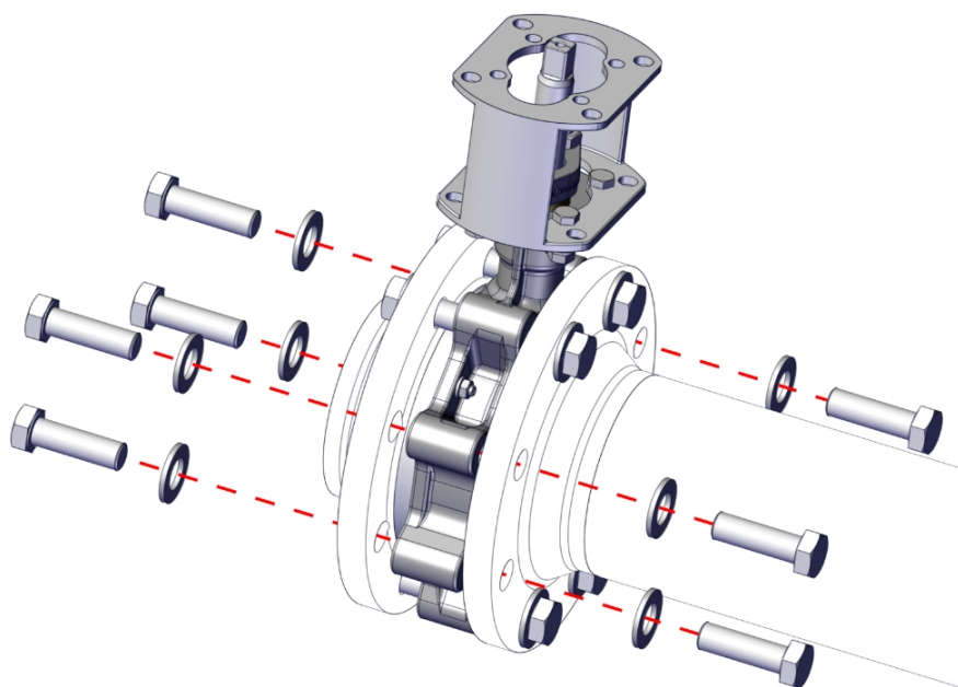
Fig. 9 : Vissage du clapet à bride
