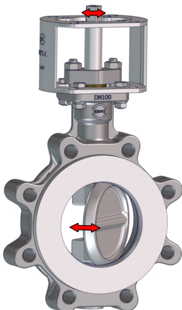
Fig. 4 : Pièces mobiles
