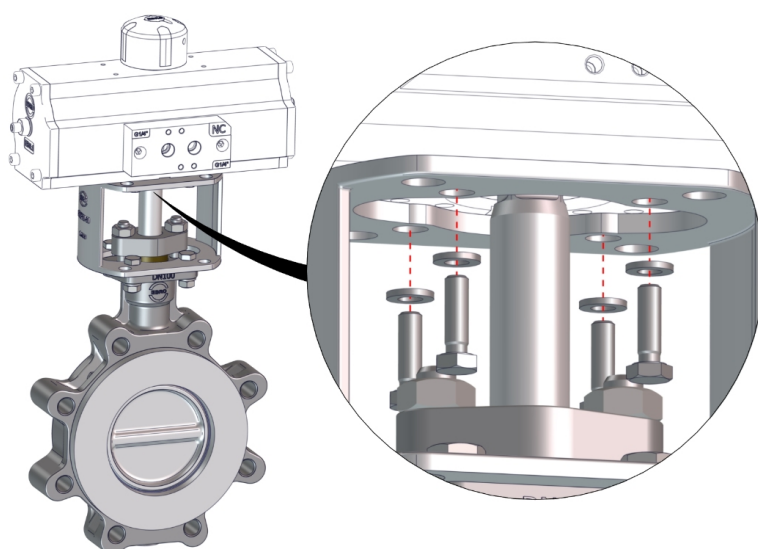
Fig. 7 : Principe de montage des composants
