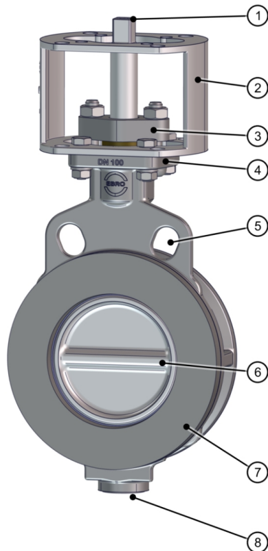
Fig. 2 : Composants
