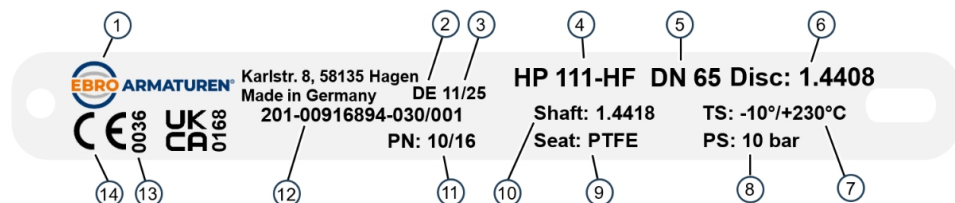
Fig. 1 : Exemple de plaque signalétique
