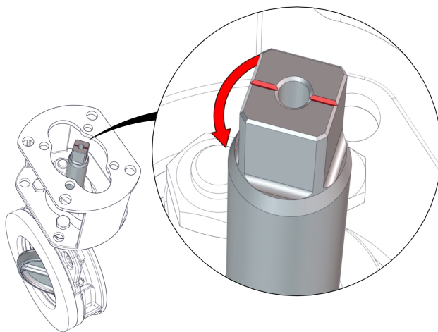
Fig. 14 : Sens d'actionnement
