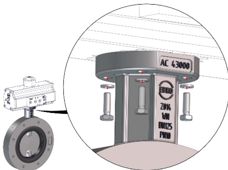
Fig. 7 : Principe de montage des composants
