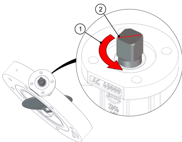
Fig. 14 : Sens d'actionnement
