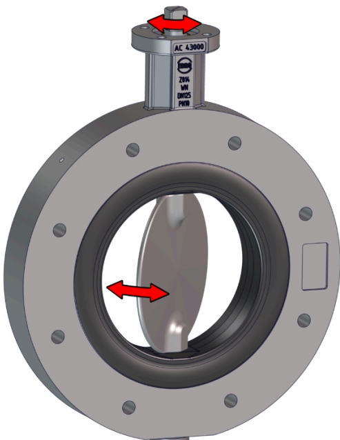
Fig. 4 : Pièces mobiles
