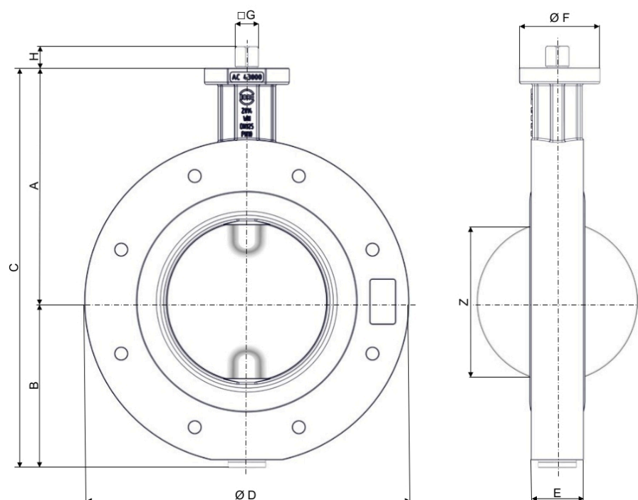
Fig. 3 : Dimensions principales Z014-WN
