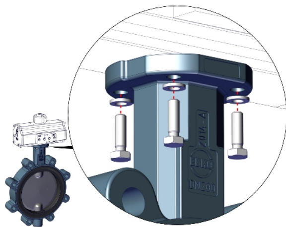
Fig. 7 : Principe de montage des composants
