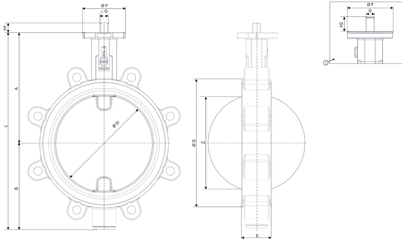
Fig. 3 : Dimensions principales Z014-B
