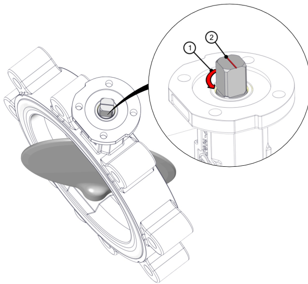
Fig. 14 : Sens d'actionnement
