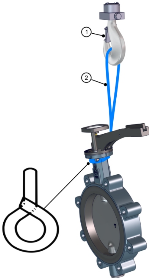
Fig. 6 : Transport par grue du clapet à bride
