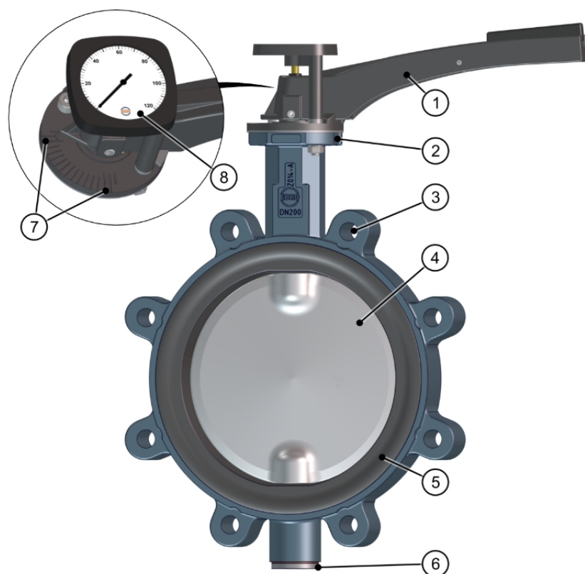
Fig. 2 : Composants
