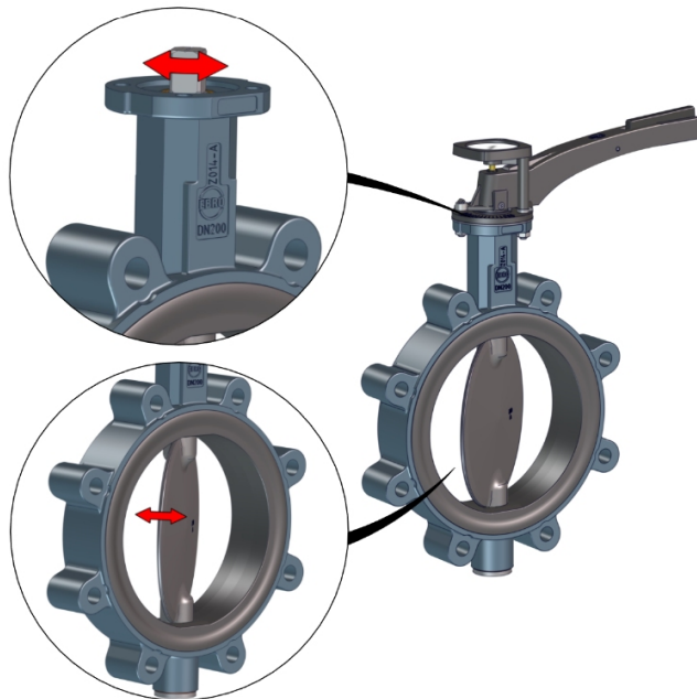
Fig. 4 : Pièces mobiles
