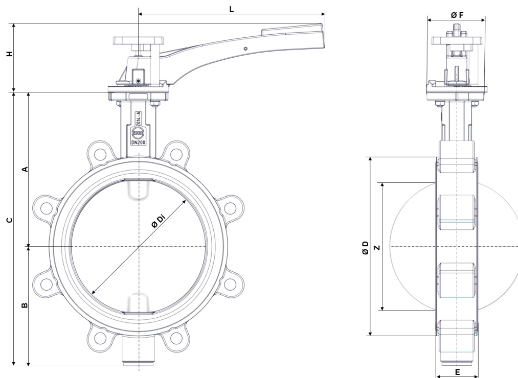
Fig. 3 : Dimensions principales Z014-A THERM
