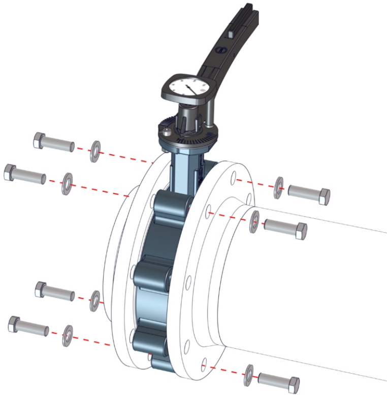
Fig. 8 : Positionnement du clapet à bride
