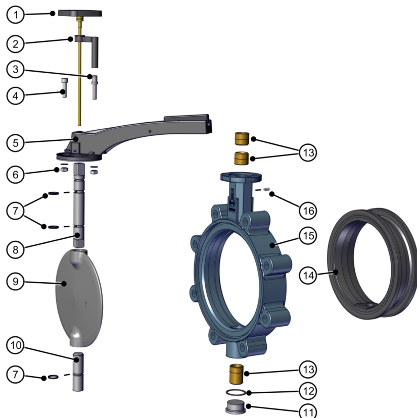
Fig. 16 : Nomenclature Z014-A THERM
