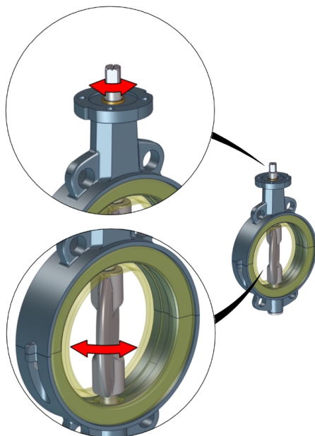
Fig. 4 : Pièces mobiles
