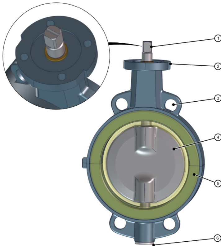
Fig. 2 : Composants
