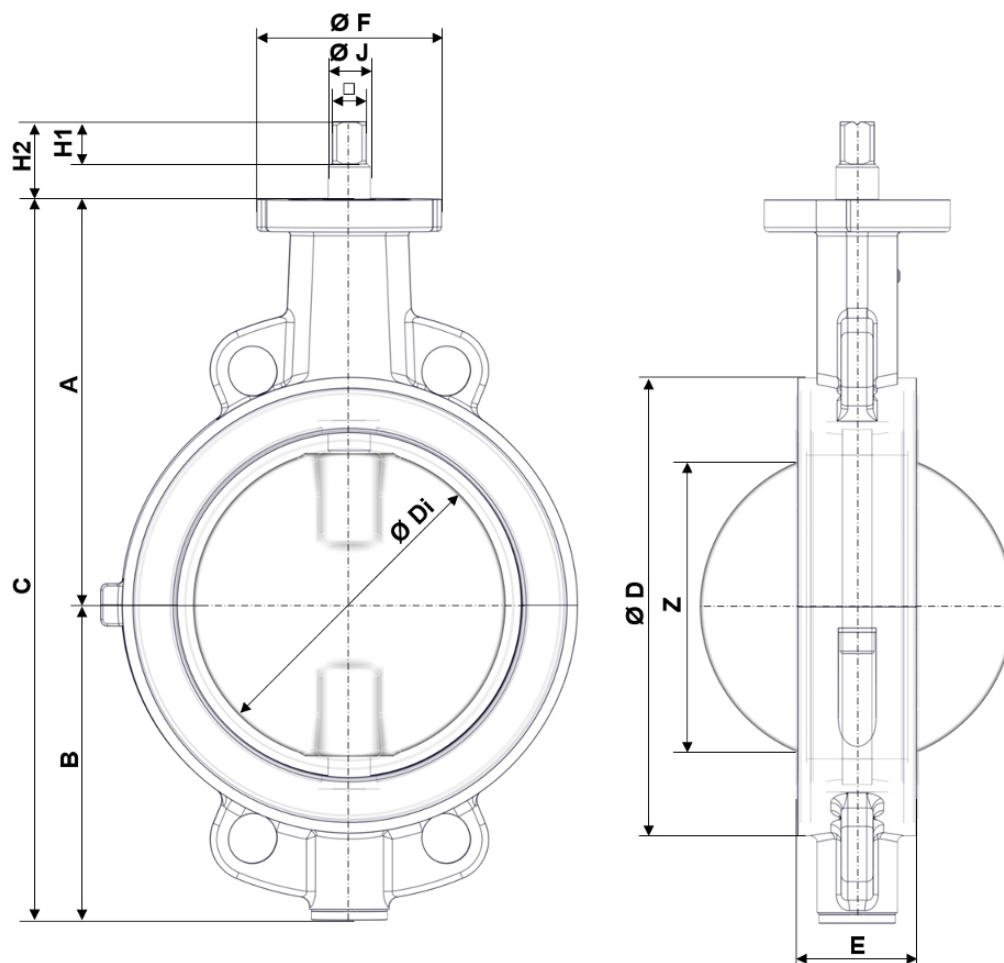
Fig. 3 : Dimensions principales Z011-GMX
