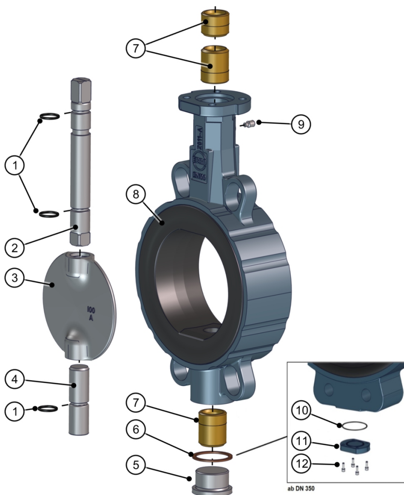
Fig. 15 : Nomenclature Z011-B arbre divisé
