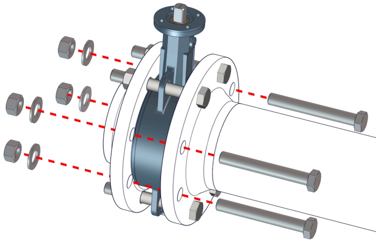
Fig. 9 : Vissage du clapet à bride intermédiaire
