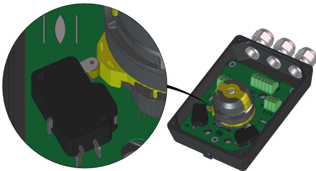
Fig. 10 : Réglage de la came « OUVERT »
