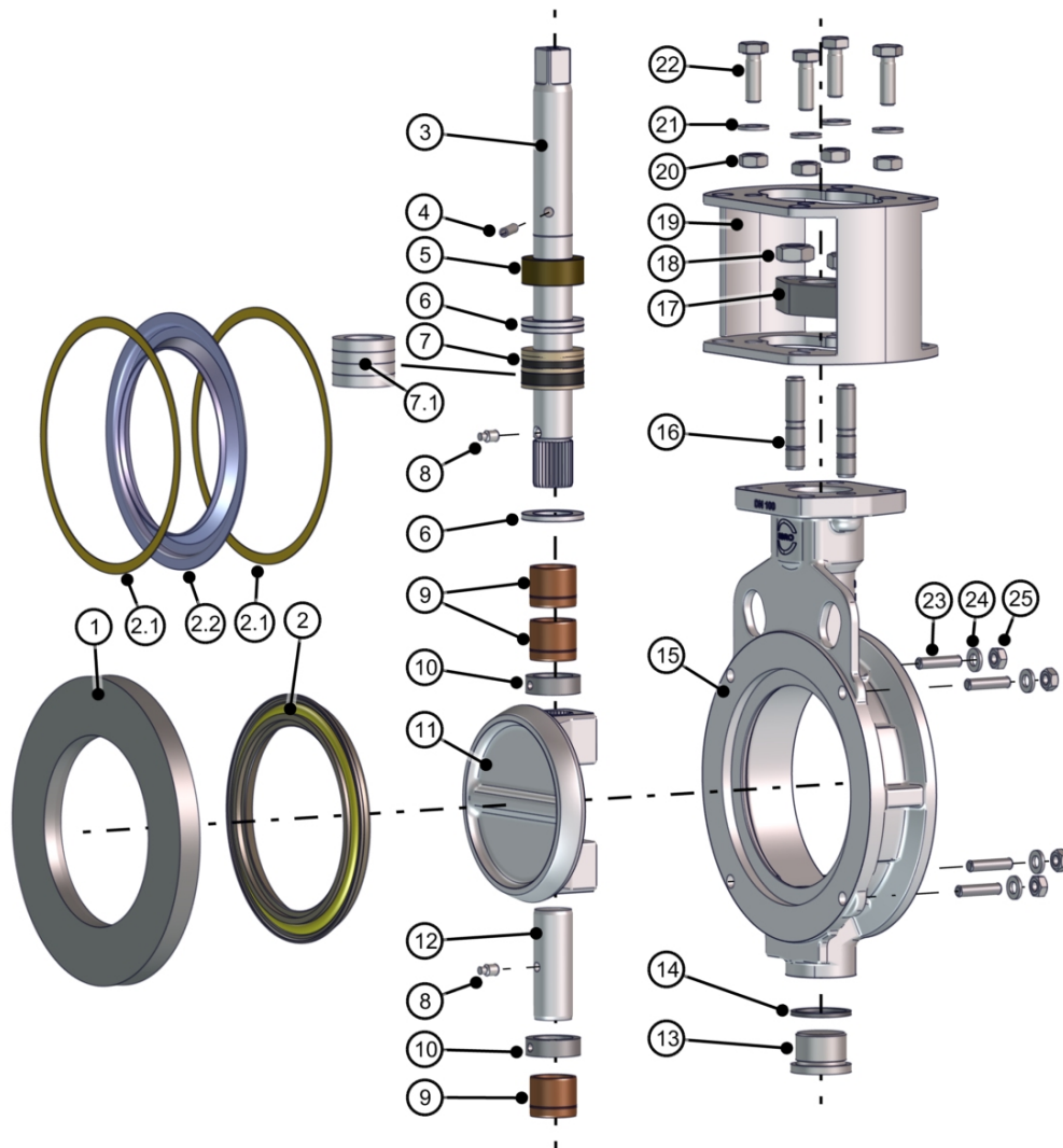
Kuva 15: Osaluettelo HP111-HF
