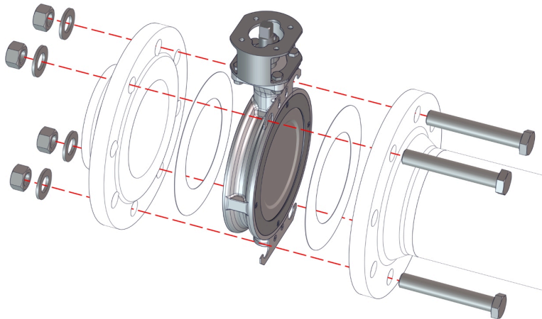
Kuva 8: Välilaipan luukun kohdistaminen
