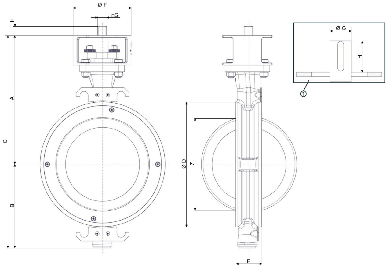
Kuva 3: Päämitat HP111
