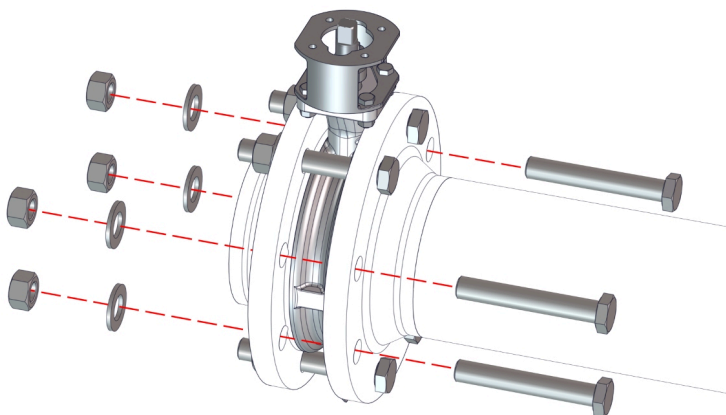
Kuva 9: Välilaipan luukun ruuvaus
