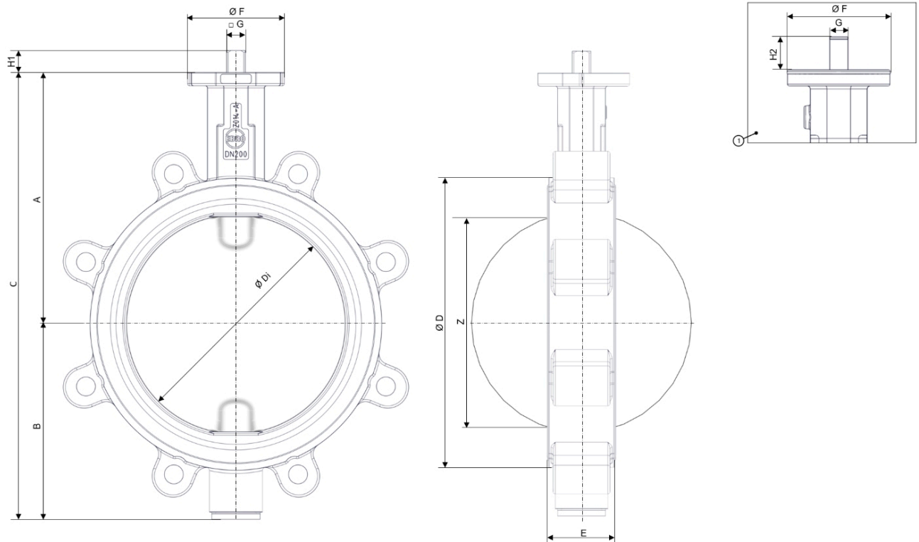
Kuva 3: Päämitat Z014-B
