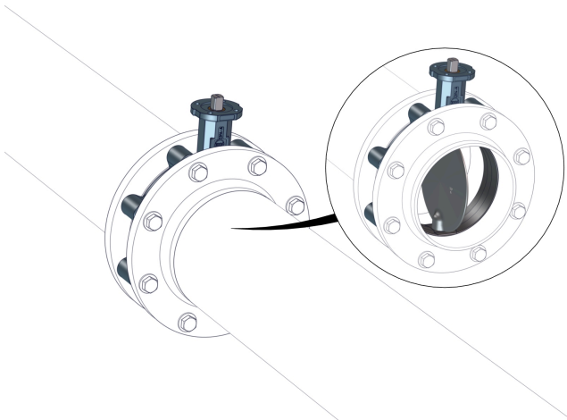
Kuva 13: Huuhteleventtiili
