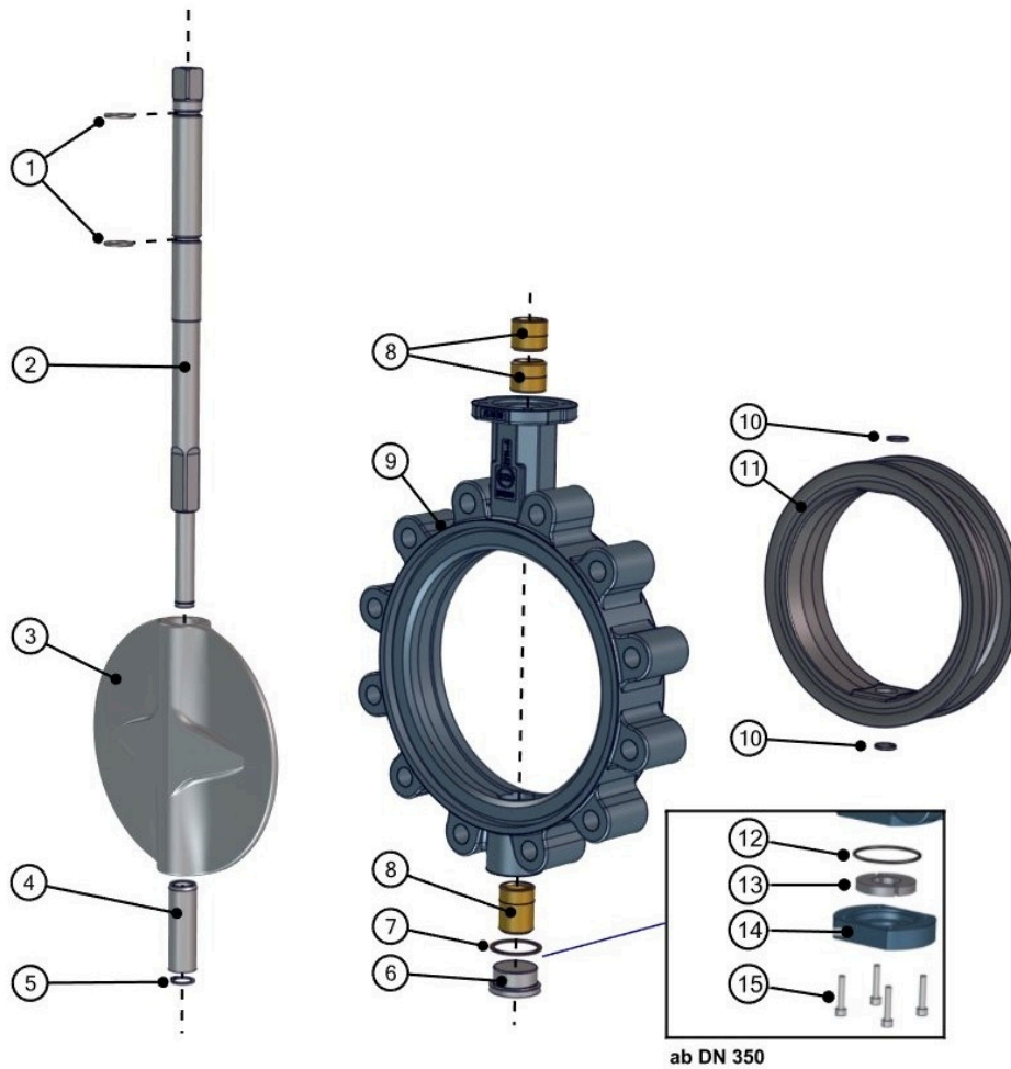
Kuva 16: Osaluettelo Z014-A TS-akseli
