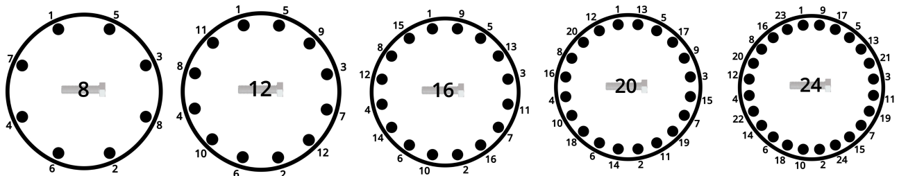
Kuva 12: Putkilaipan ruuvien kiristysjärjestys
