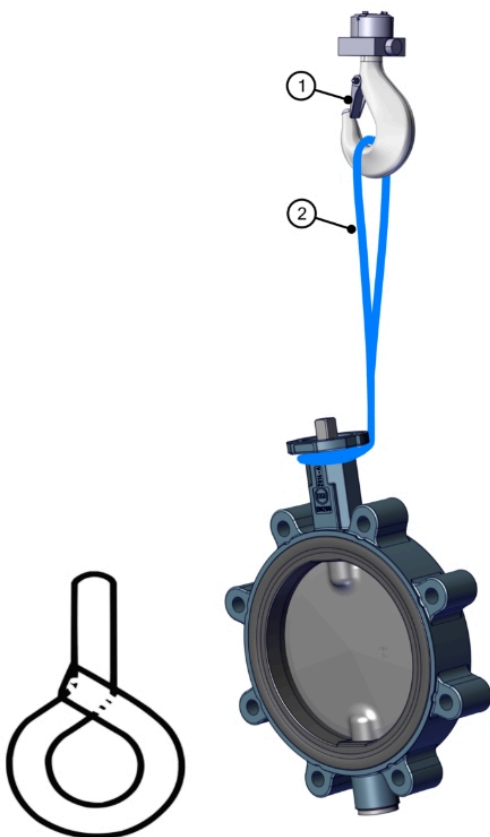
Kuva 6: Laippaläpän nostaminen
