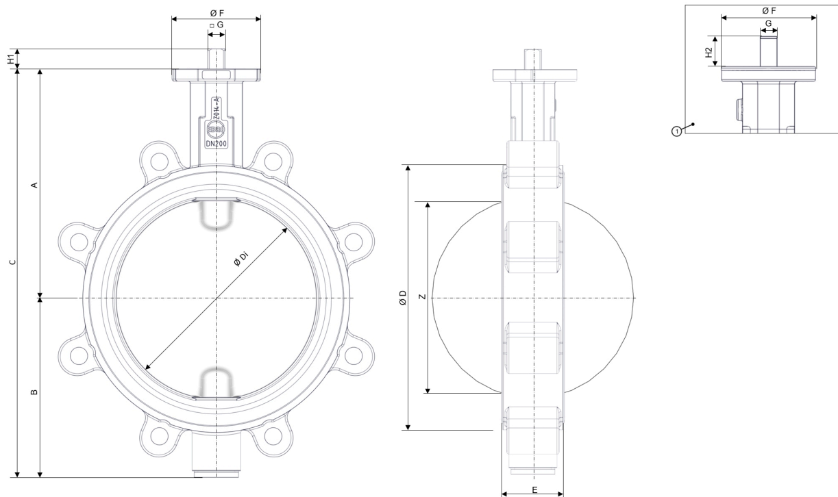
Kuva 3: Päämitat Z014-A
