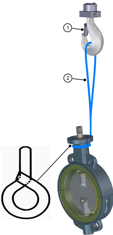
Kuva 6: Välilaitan luukun nostaminen
