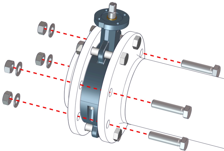
Kuva 9: Välilaipan luukun ruuvaus
