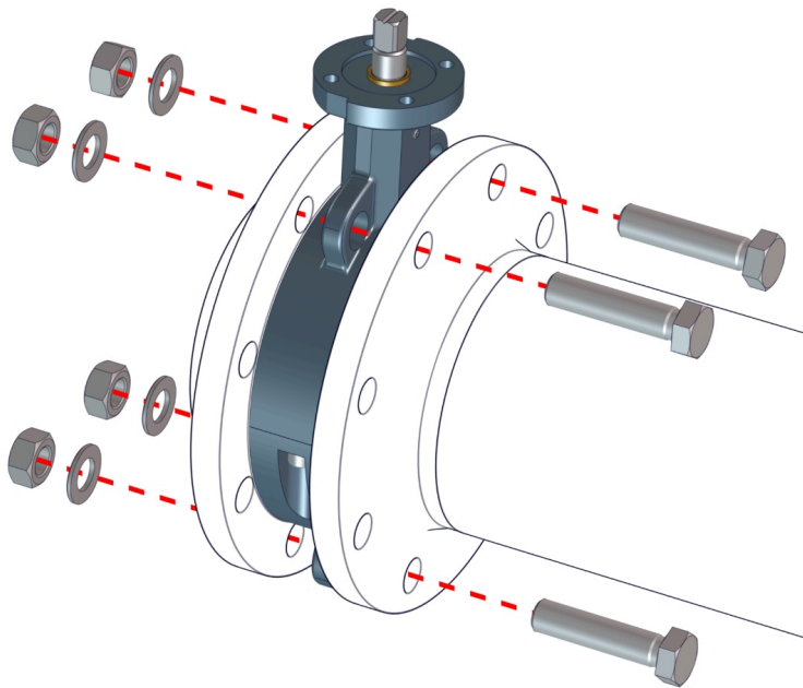
Kuva 8: Välilaipan luukun kohdistaminen
