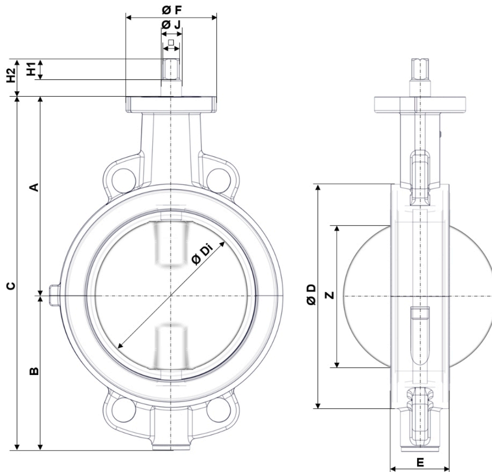
Kuva 3: Päämitat Z011-GMX
