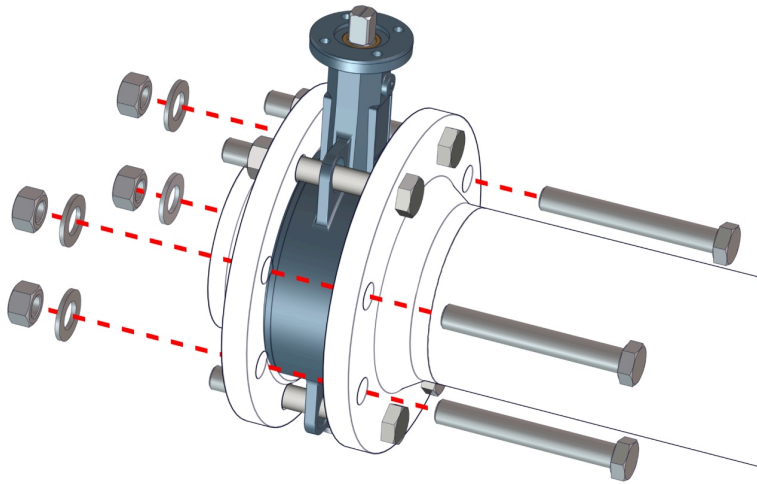
Kuva 9: Välilaipan luukun ruuvaus
