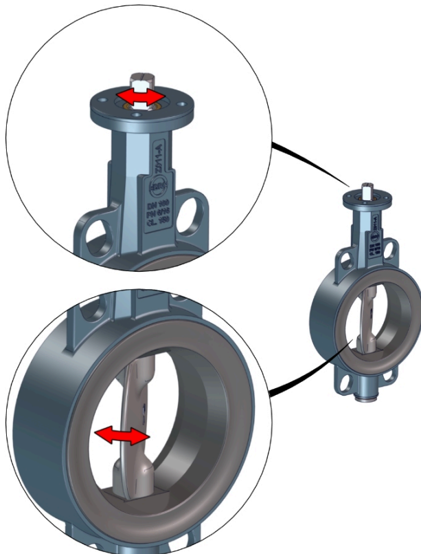
Kuva 4: Liikkuvia osia
