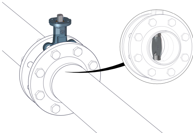
Kuva 13: Huuhtelevä putki
