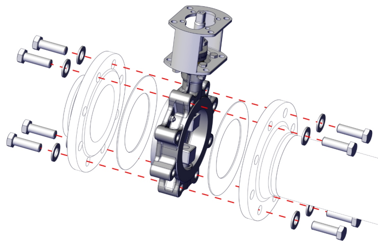
Joonis 8: Äärikuga klapi positsioneerimine
