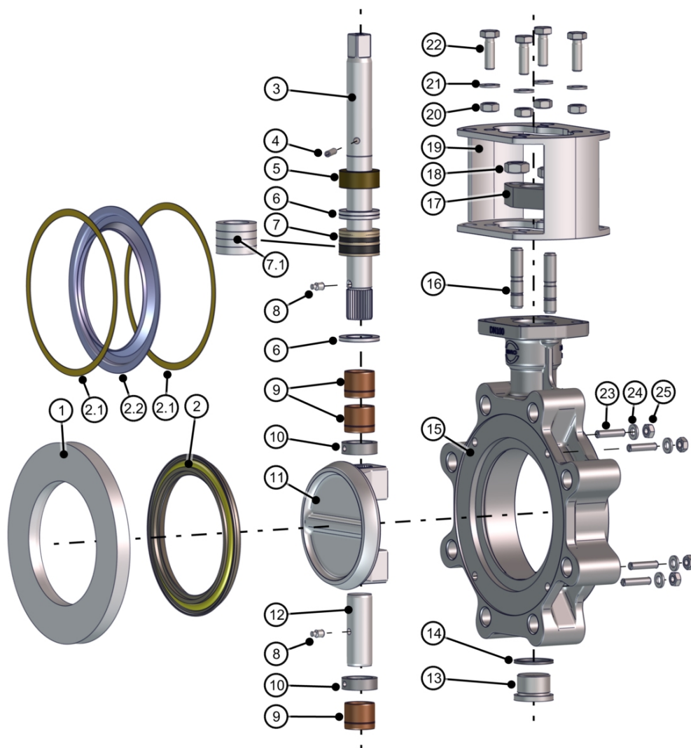
Joonis 15: Osade loetelu HP114-HF
