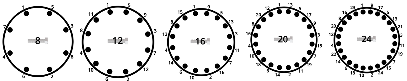
Joonis 12: Toru äärikukruvi kinnikeeramise järjekord
