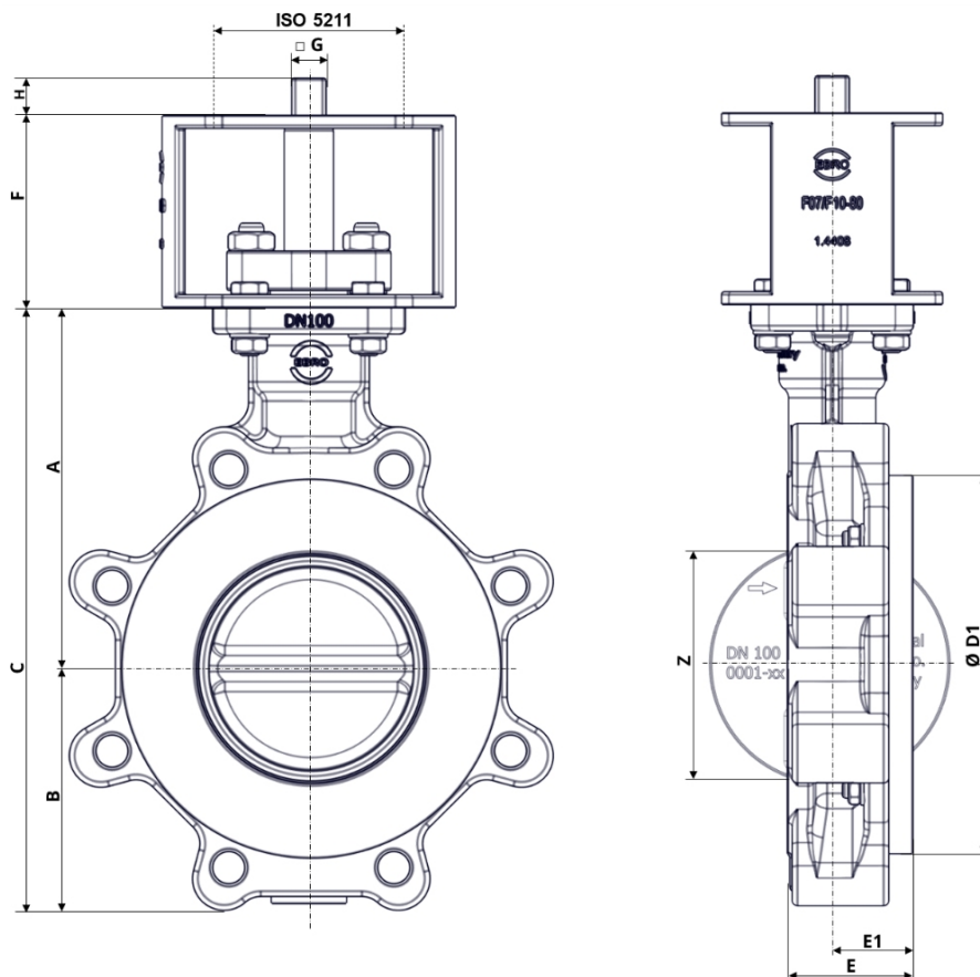
Joonis 3: Põhimõõtmed HP114-HF
