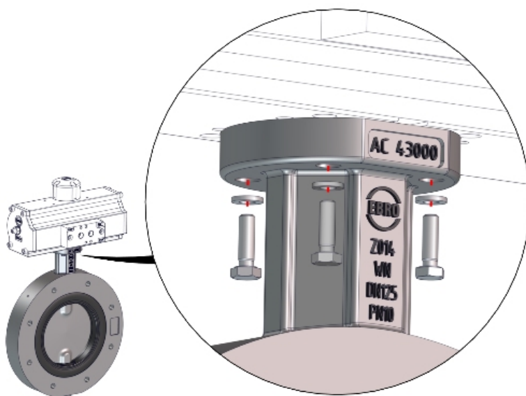
Joonis 7: Komponentide monteerimise põhimõte
