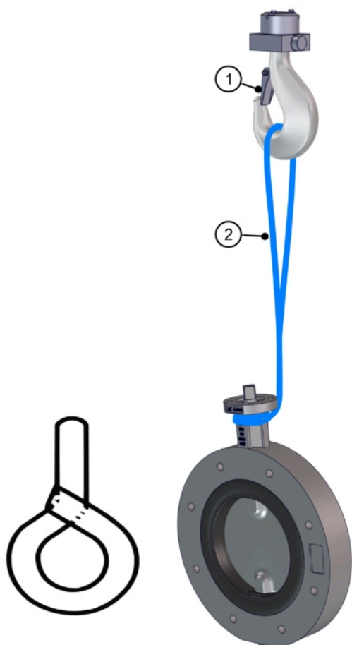
Joonis 6: Täisäärikuga klapi kraanaga tõstmine
