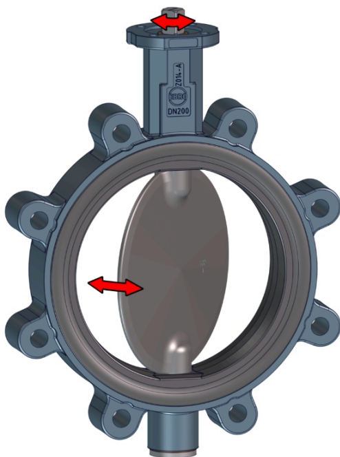
Joonis 4: Liikuvad osad
