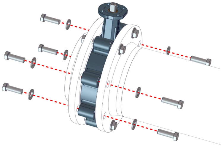
Joonis 9: Äärikuga klapi kinnikruvimine
