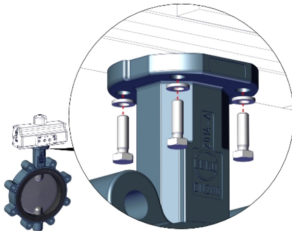
Joonis 7: Komponentide monteerimise põhimõte
