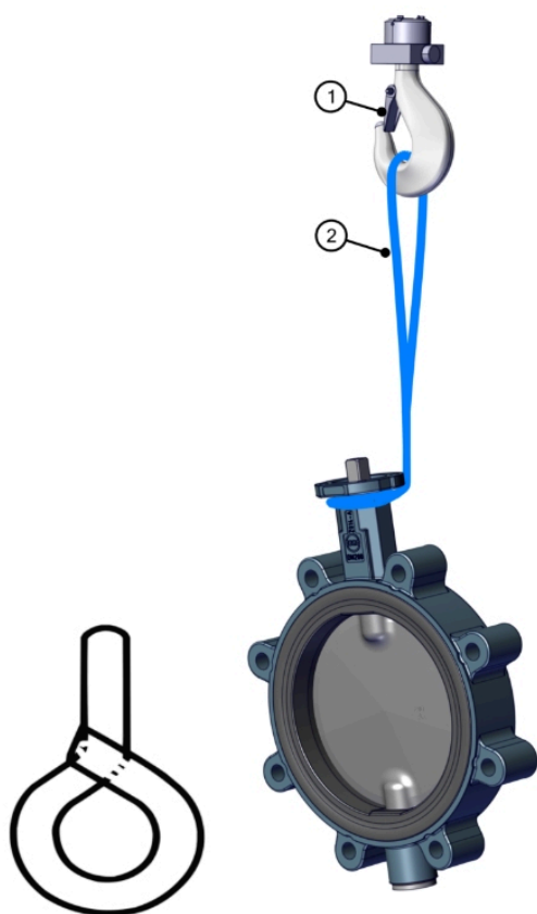
Joonis 6: Äärikuga klapi kraanaga tõstmine
