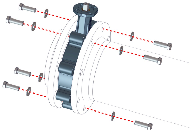
Joonis 8: Äärikuga klapi positsioneerimine
