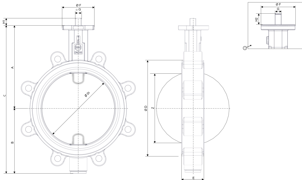
Joonis 3: Põhimõõtmed Z014-A
