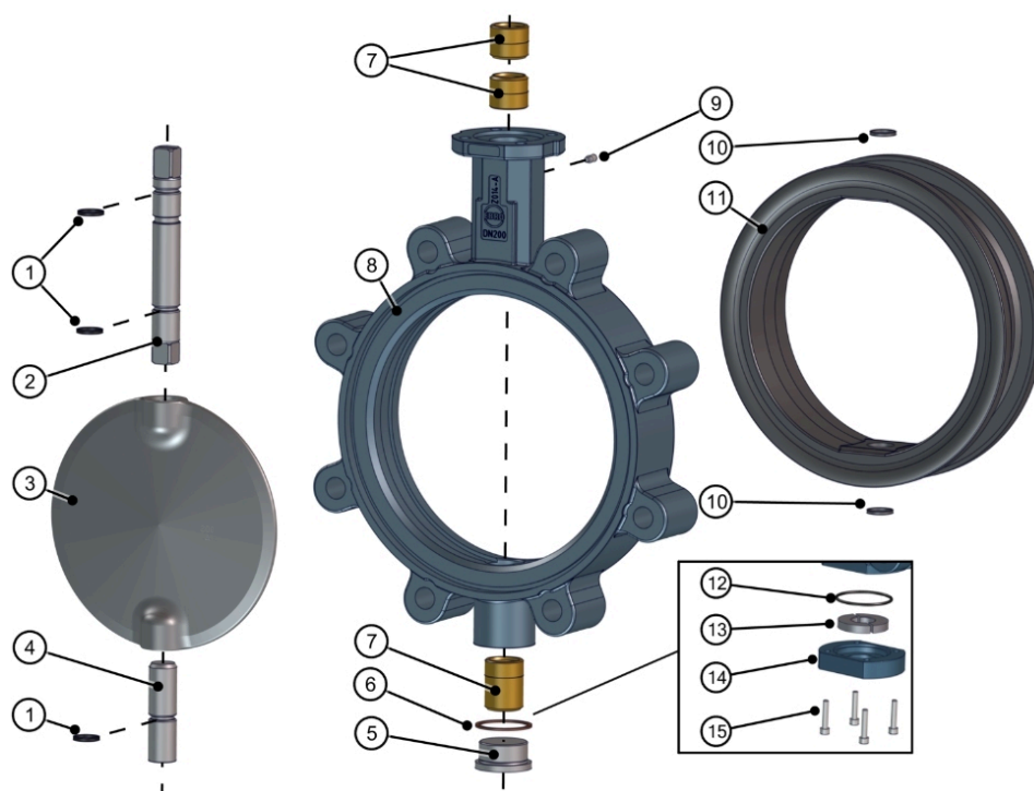
Joonis 15: Osade loetelu Z014-A
