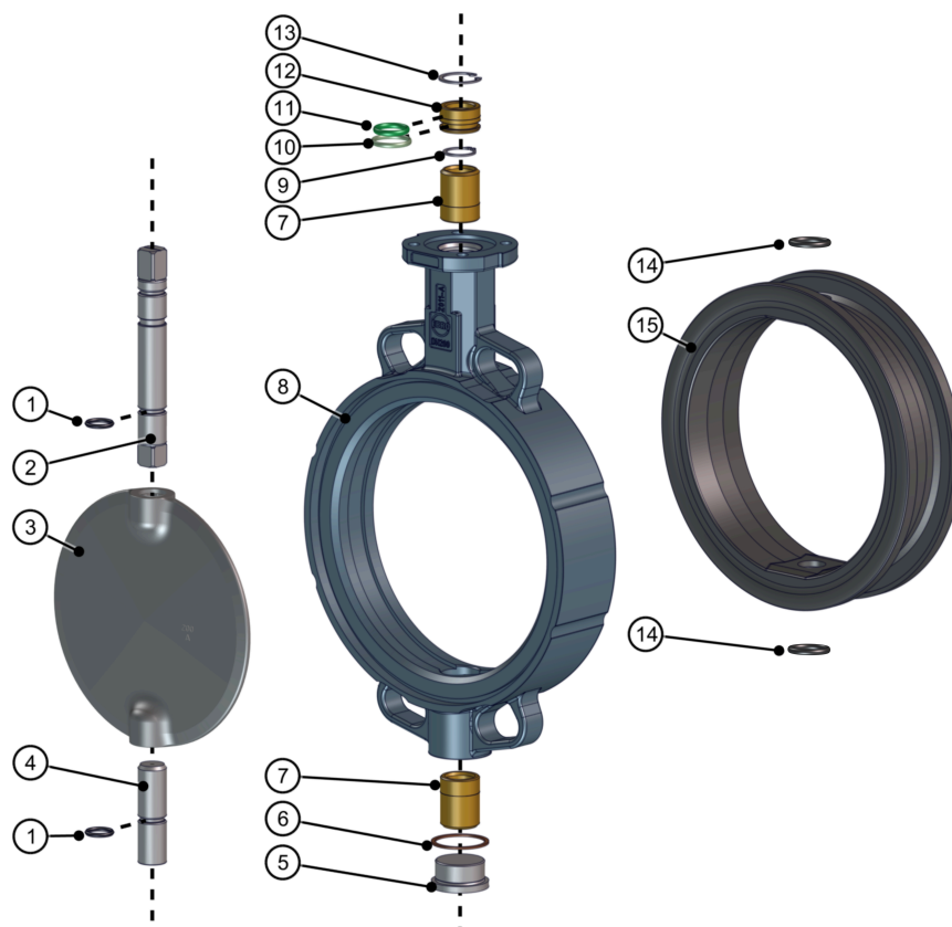
Joonis 17: Osade loetelu täppisvalu-ketas, 2 võlliga
