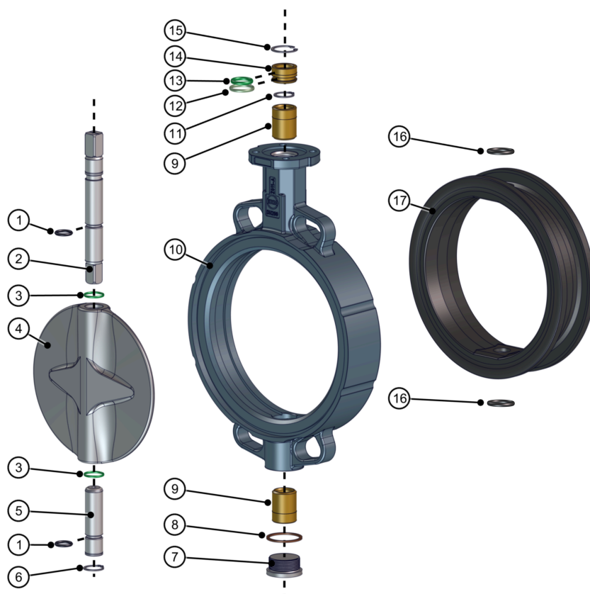
Joonis 19: Osade loetelu TS-ventiiliketas, 2 völliiga
