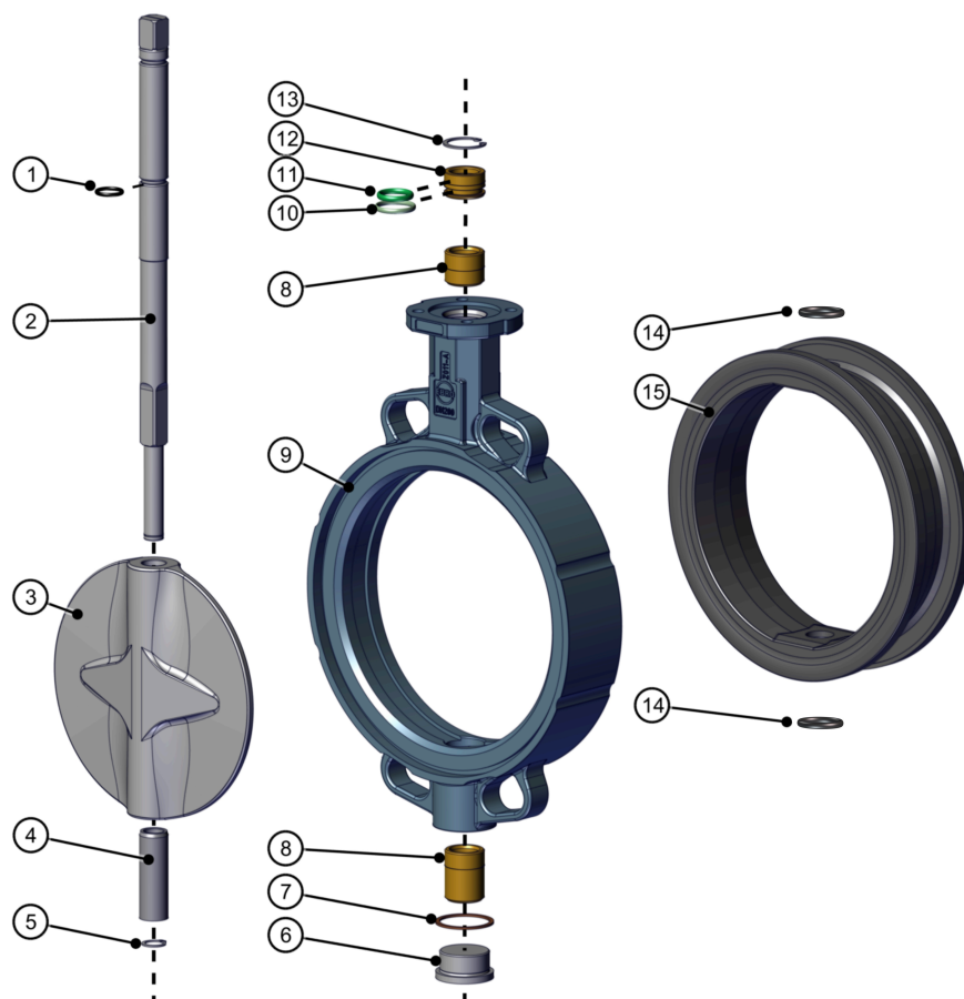
Joonis 18: Osade loetelu TS-ventiiliketas, 1 võlliga
