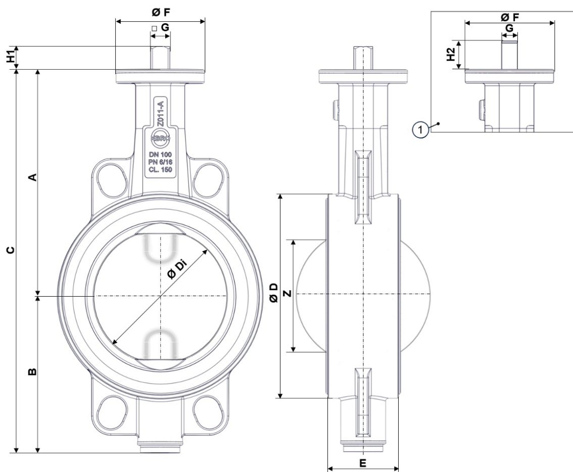
Joonis 3: Põhimõõtmed Z011-AS
