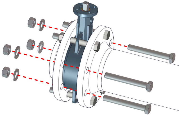
Joonis 9: Vaheäärikuga klapi kinnikruvimine
