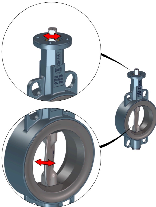
Joonis 4: Liikuvad osad
