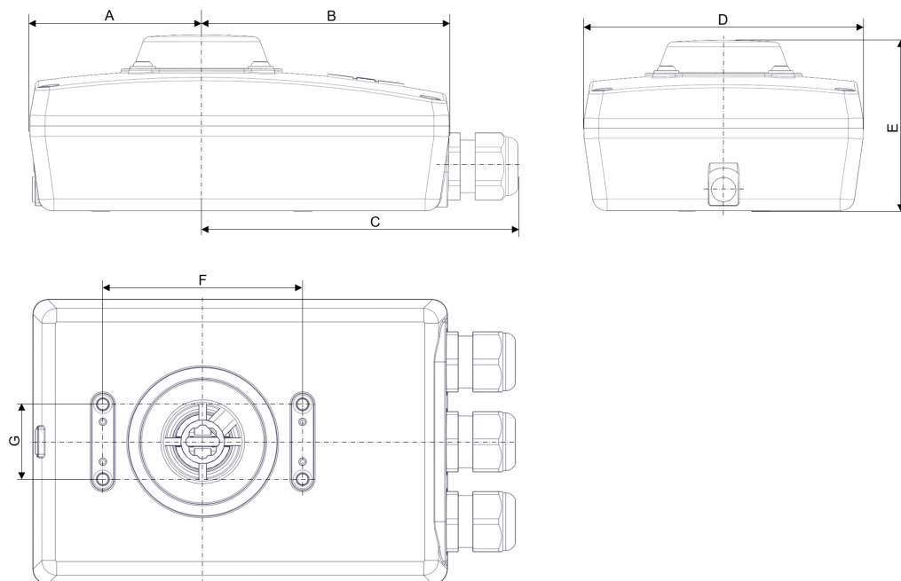
Joonis 4: Mõõtmed
