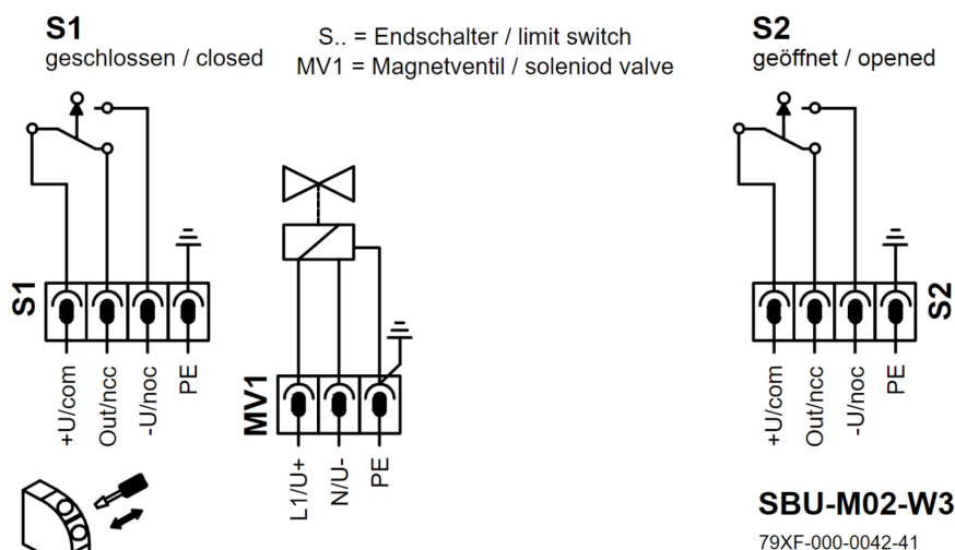
Joonis 7: Elektriskeem SBU Basic
