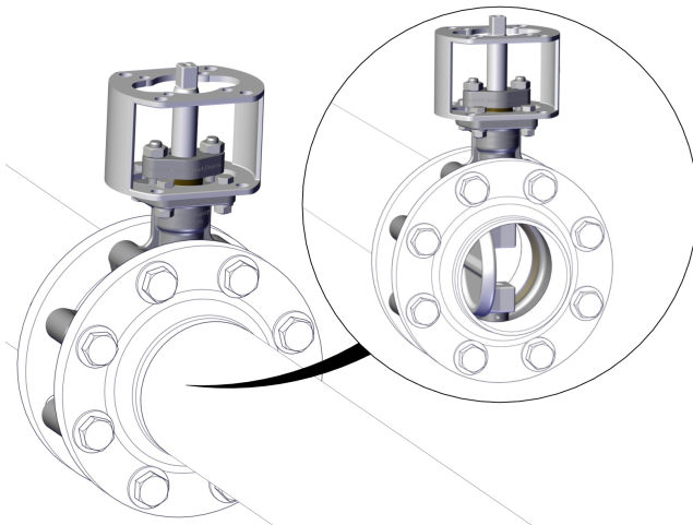
Afb. 13: Buis spoelen
