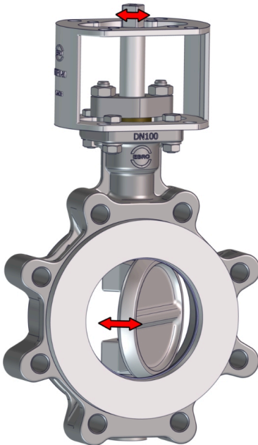
Afb. 4: Bewegende onderdelen
