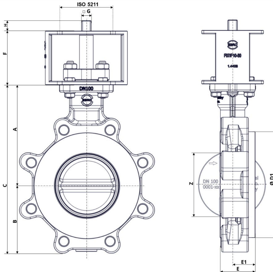
Afb. 3: Hoofdafmetingen HP114-HF
