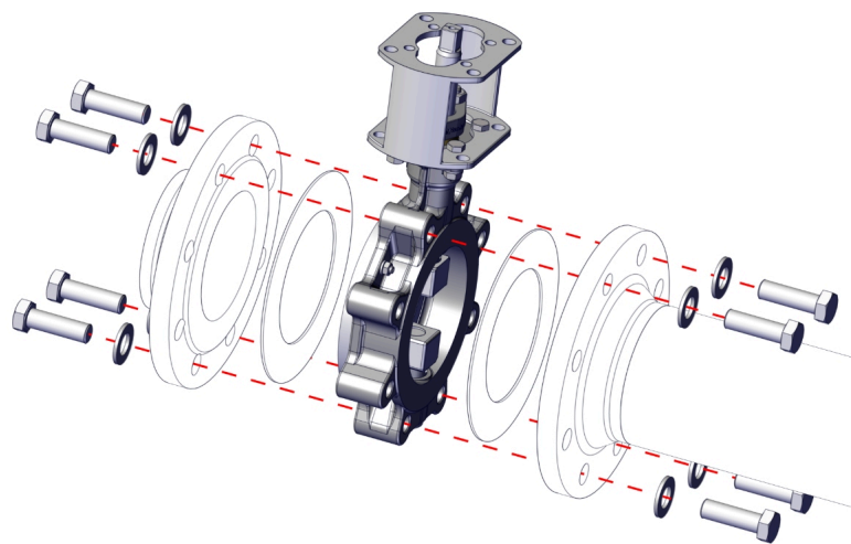
Afb. 8: Afsluitklep met aansluitflenzen positioneren
