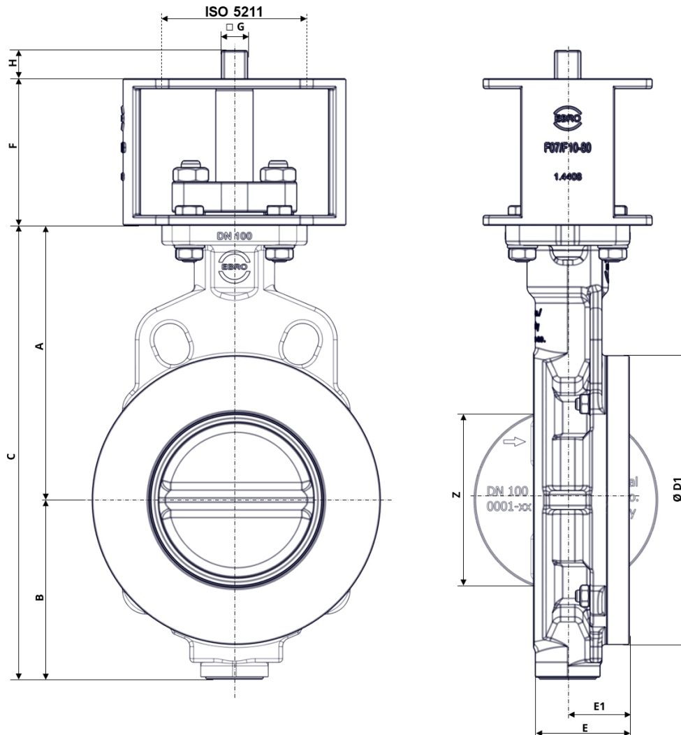
Afb. 3: Hoofdafmetingen HP111-HF
