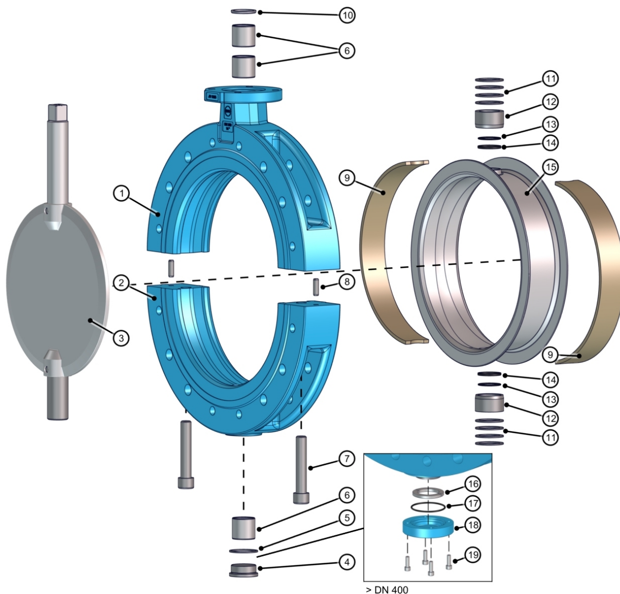
Afb. 15: Stuklijst T212-A
