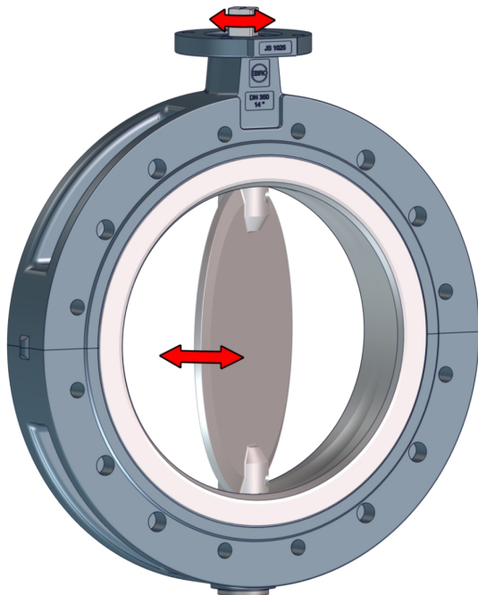
Afb. 4: Bewegende onderdelen
