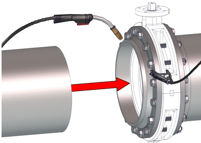
Afb. 10: Buis met flens lassen
