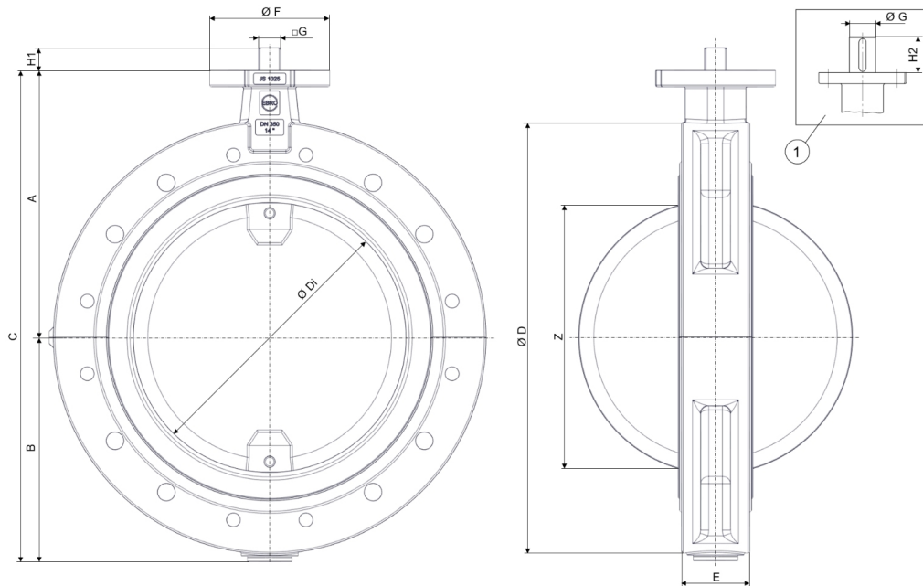
Afb. 3: Hoofdafmetingen T212-A
