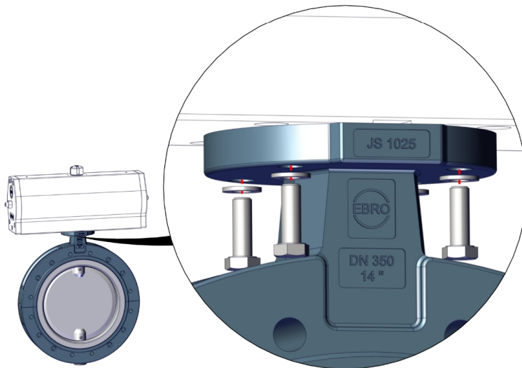
Afb. 7: Principe van componenten monteren
