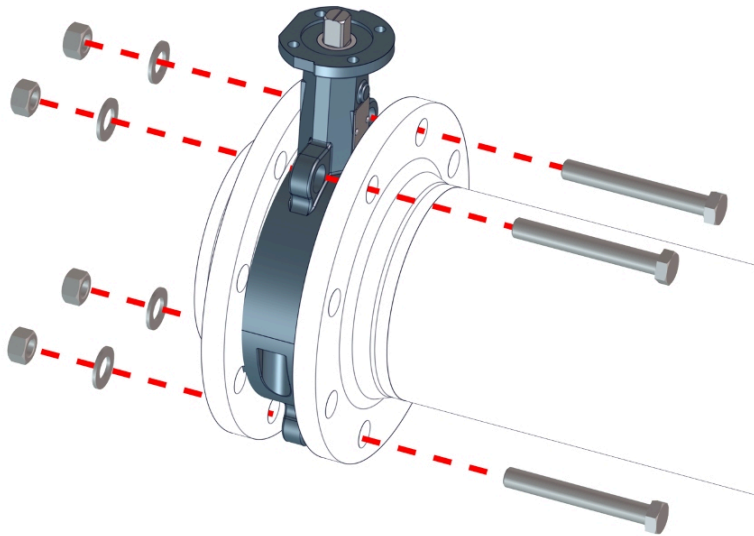
Afb. 8: Zwischenflanschklappe positionieren
