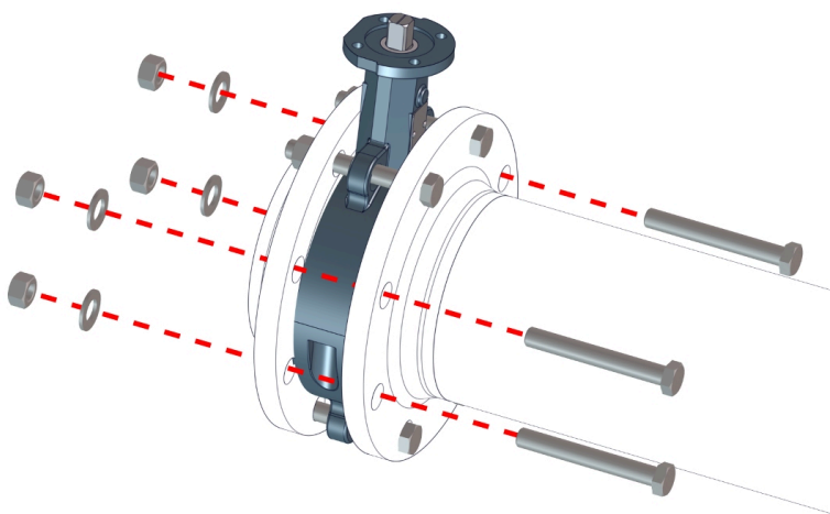
Afb. 9: Zwischenflanschklappe verschrauben
