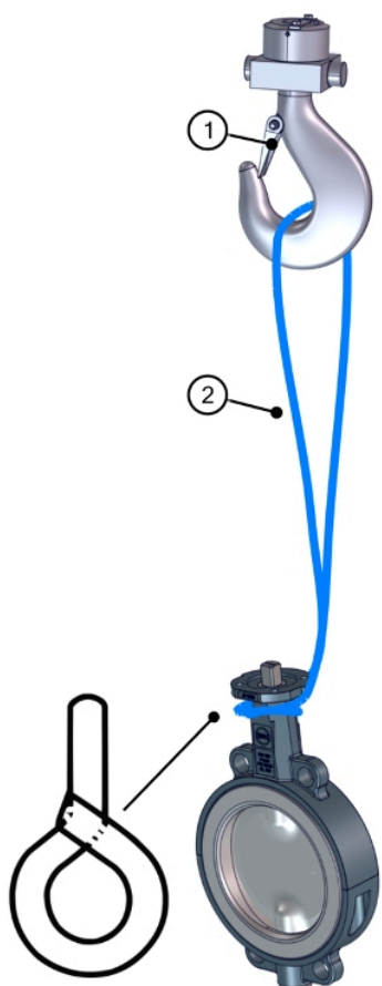
Afb. 6: Zwischenflanschklappe kranen
