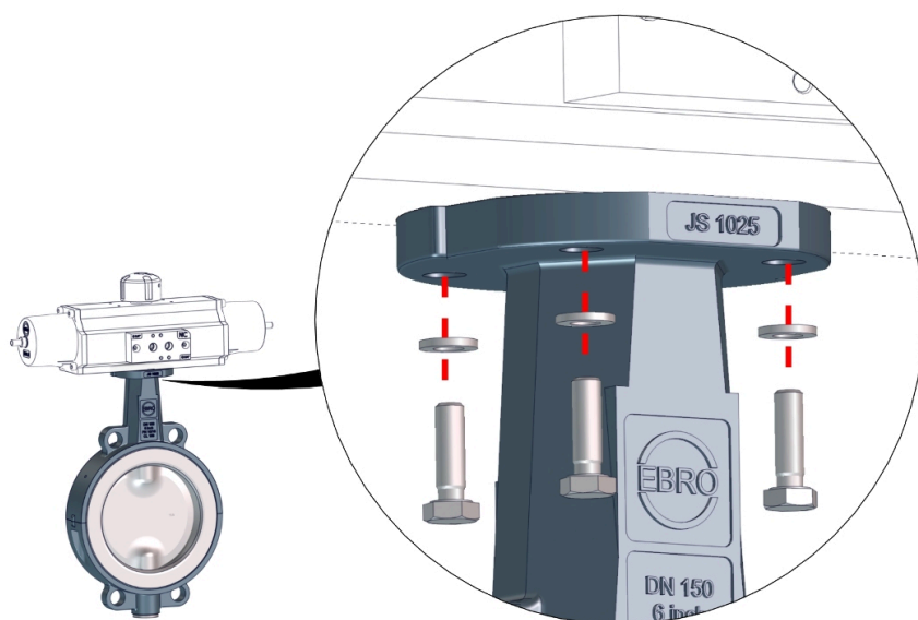
Afb. 7: Prinzip Componenten monteren
