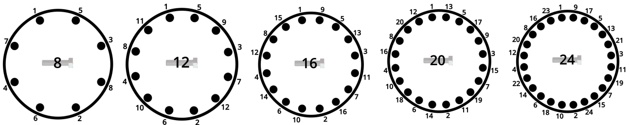
Afb. 12: Volgorde van buisflensverbinding
