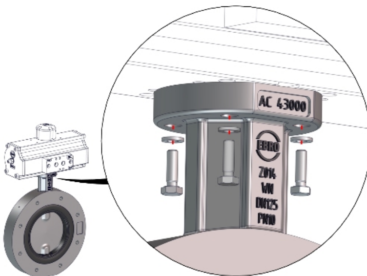
Afb. 7: Principe van componenten monteren
