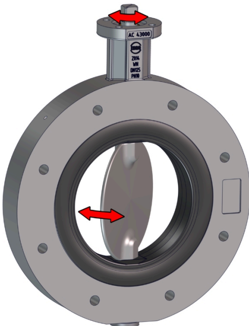
Afb. 4: Bewegende onderdelen
