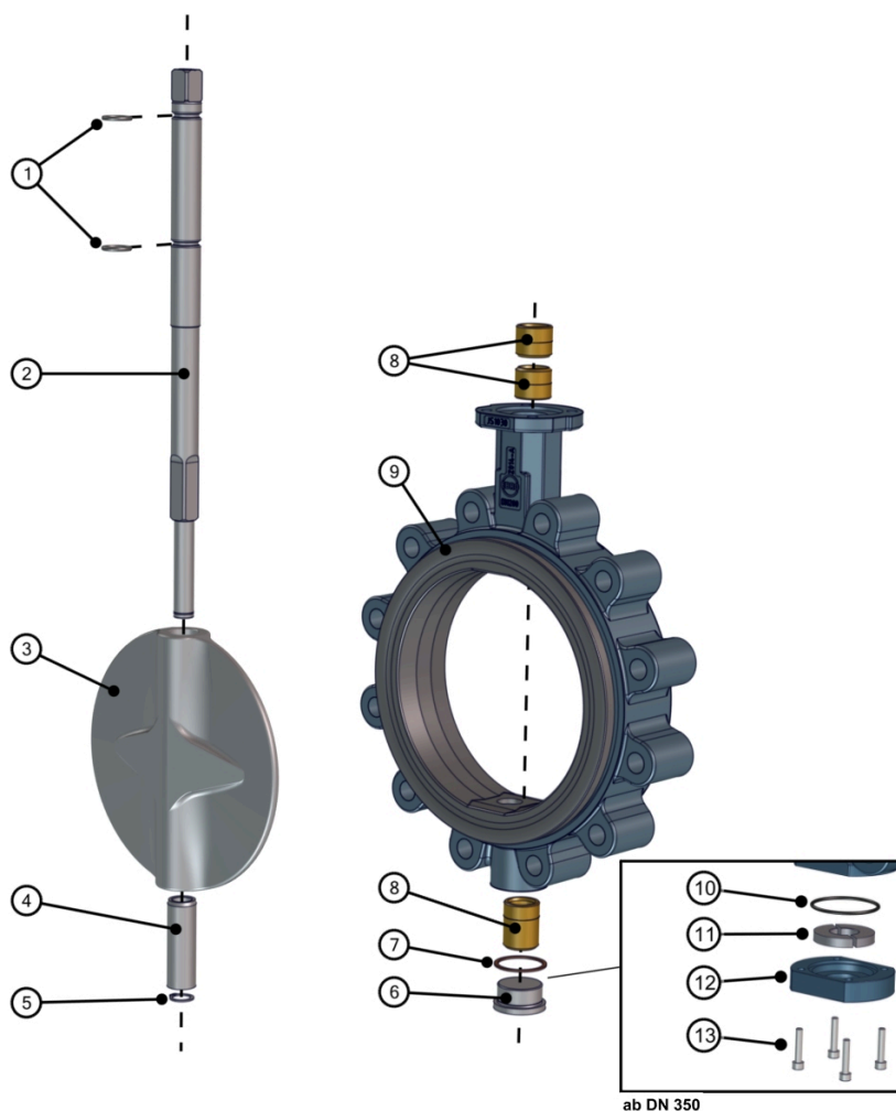
Afb. 16: Stuklijst Z14-B TS-as
