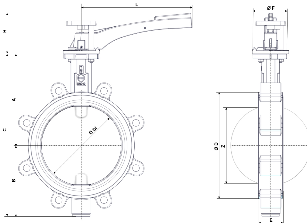
Afb. 3: Hoofdafmetingen Z14-A THERM
