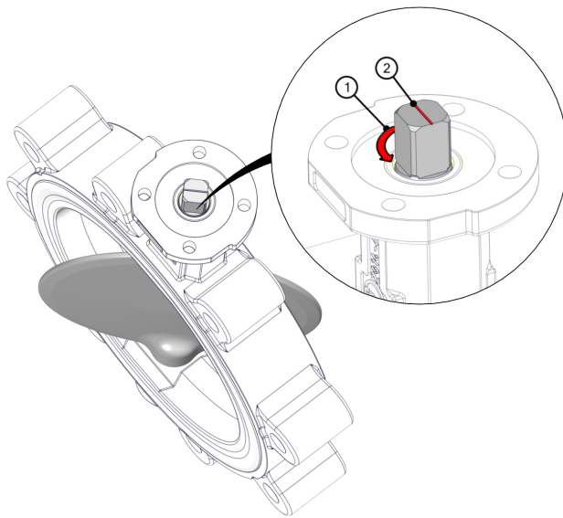
Afb. 14: Bedieningsrichting
