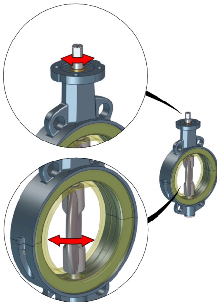
Afb. 4: Bewegende onderdelen
