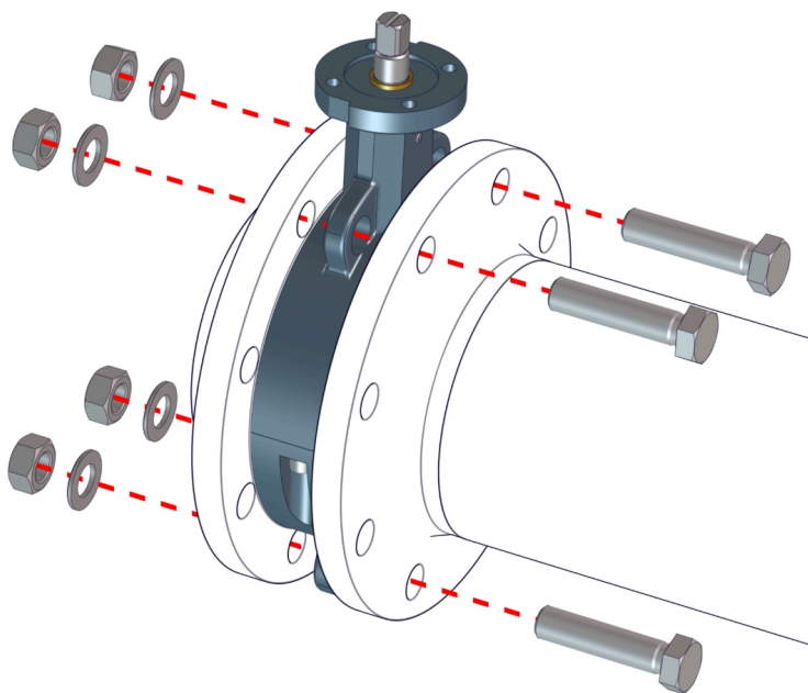
Afb. 8: Tussenflensklep positioneren
