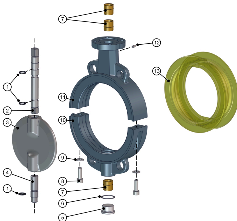
Afb. 15: Stuklijst Z011-GMX
