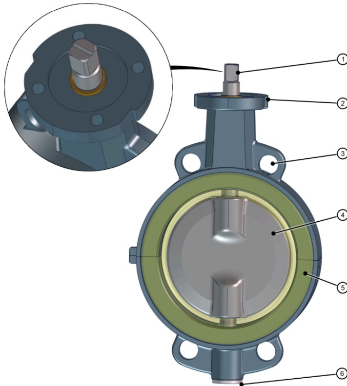
Afb. 2: Componenten
