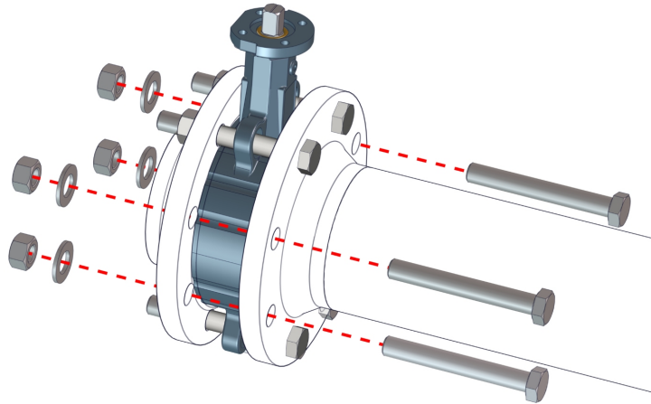
Afb. 9: Tussenflensklep vastschroeven
