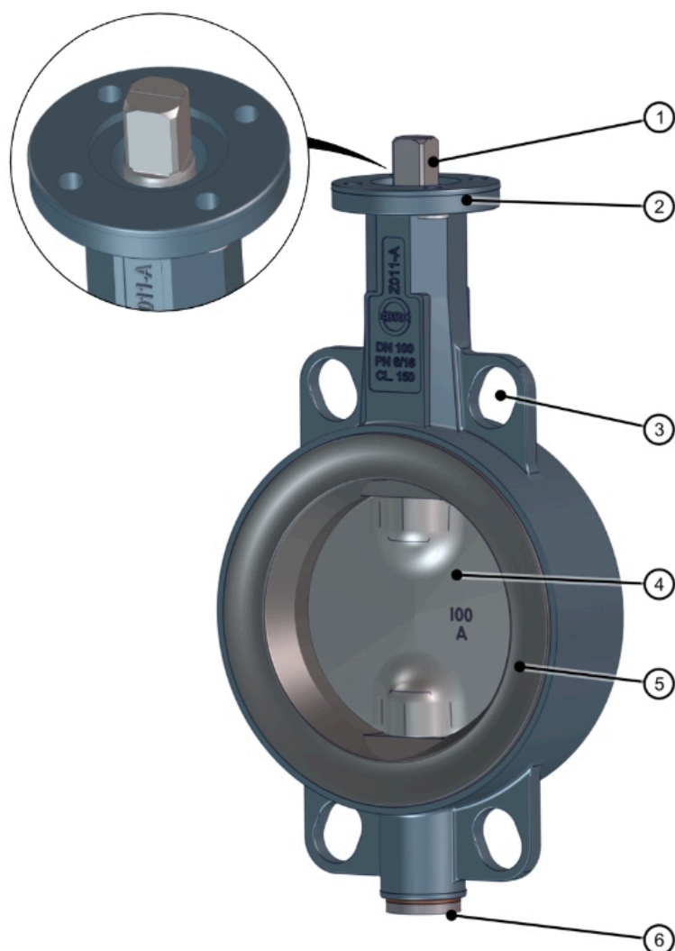
Afb. 2: Componenten
