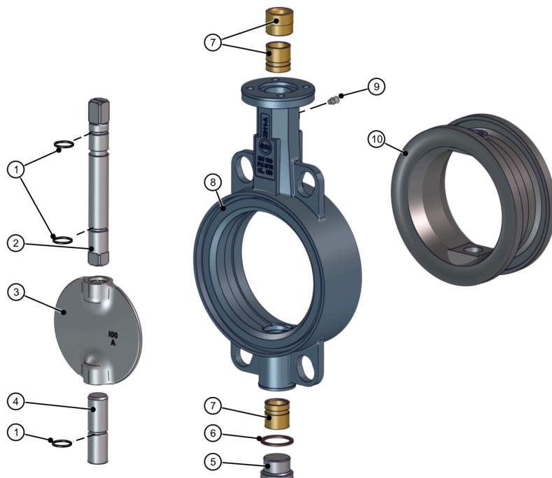
Afb. 15: Stuklijst Z011-AS
