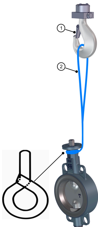
Afb. 6: Tussenflensklep kranen
