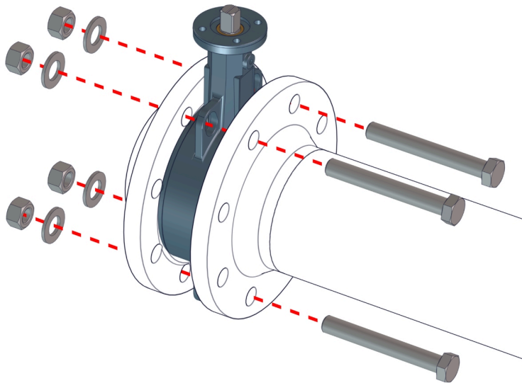
Afb. 8: Tussenflensklep positioneren
