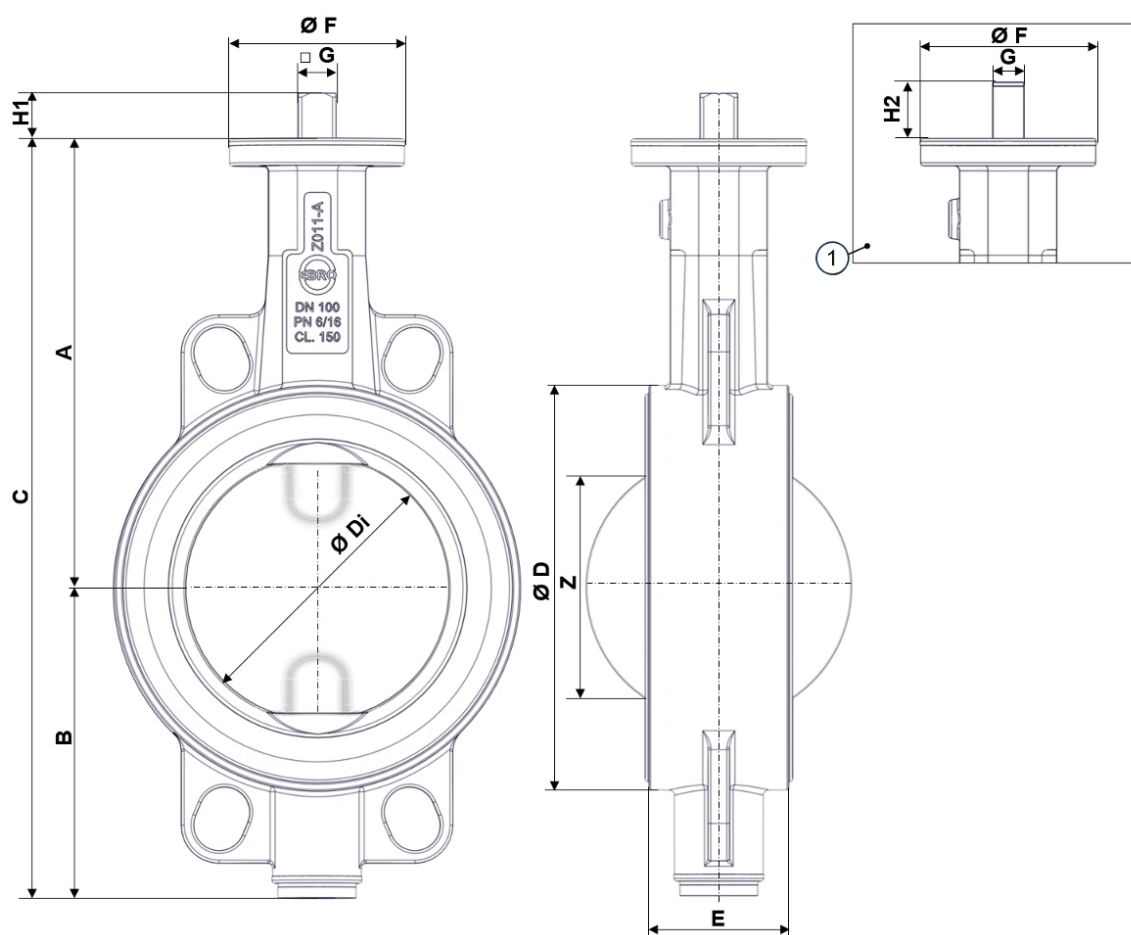
Afb. 3: Hoofdafmetingen Z011-AS
