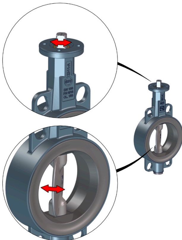
Afb. 4: Bewegende onderdelen
