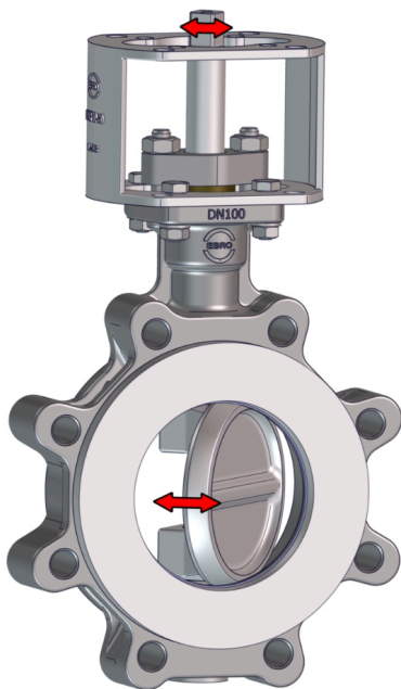
Figur 4: Bevægelige dele
