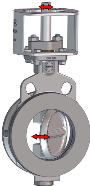
Figur 4: Bevægelige dele
