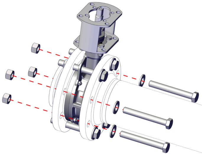
Figur 9: Skru mellemflangeklappen fast
