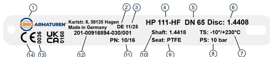
Figur 1: Eksempel-typeskilt
