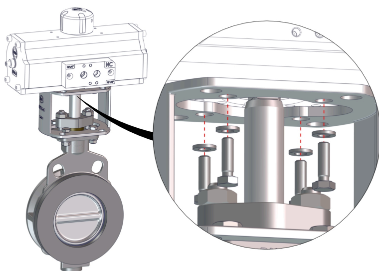
Figur 7: Princip monter komponenterne
