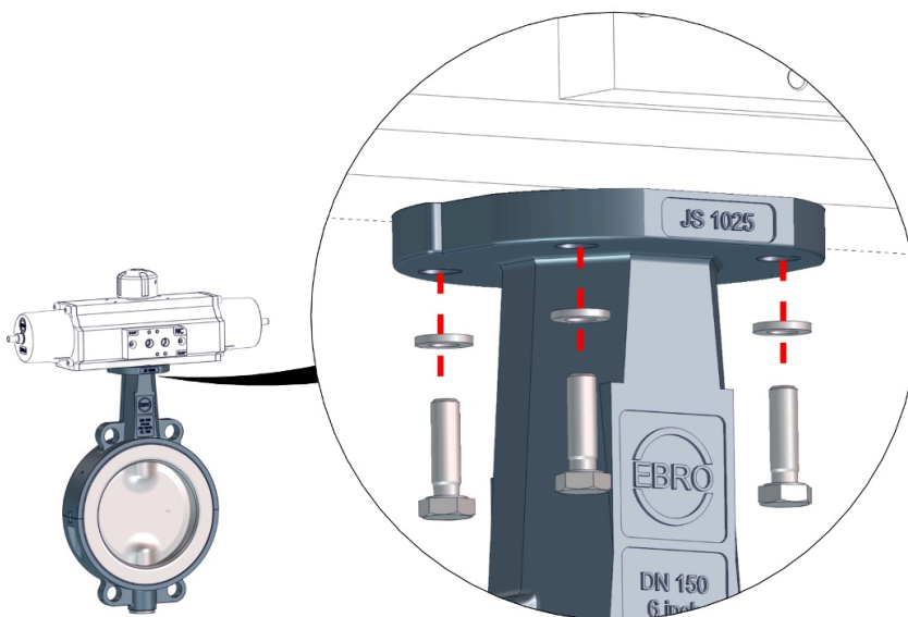
Figur 7: Prinzip Komponentens monterien
