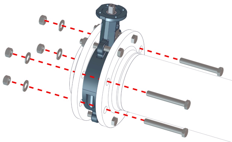
Figur 9: Zwischenflanschklappe verschrauben
