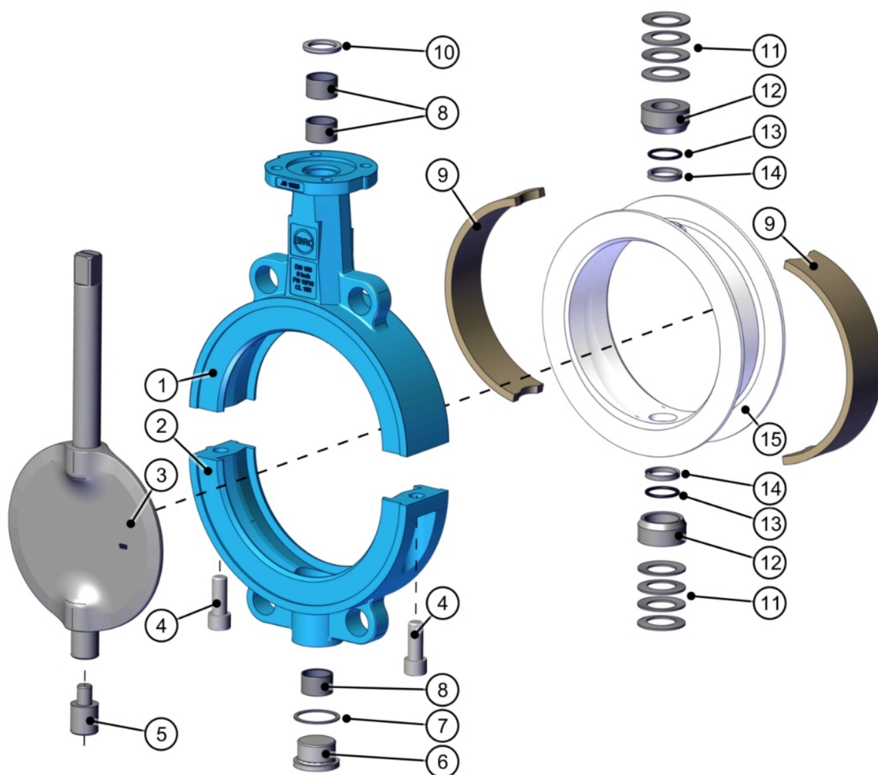
Figur 16: Stückliste T211-A ab DN40
