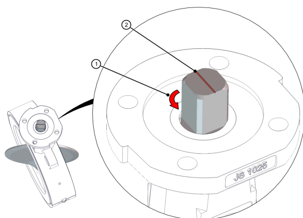
Figur 14: Betätigungsrichtung
