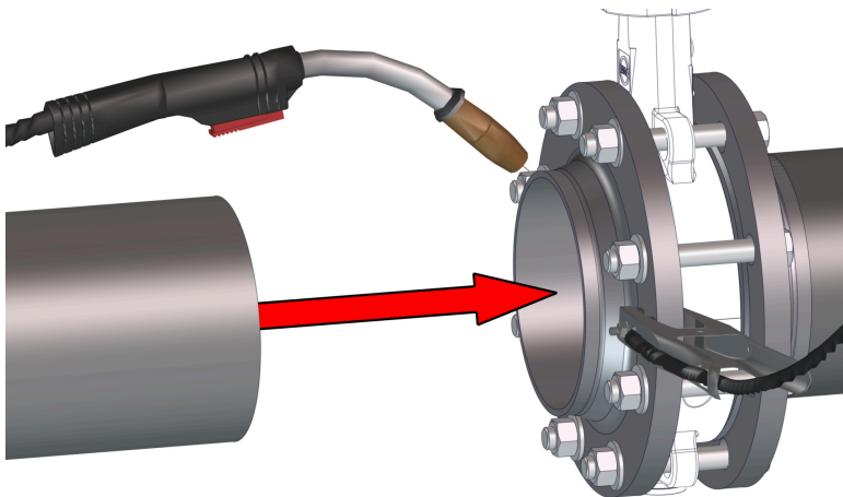
Figur 10: Rohr mit Flansch verschweißen
