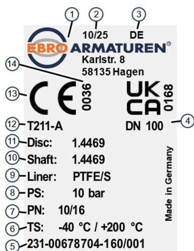
Figur 1: Eksempel typeskilt
