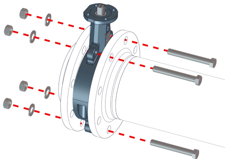
Figur 8: Zwischenflanschklappe positionieren
