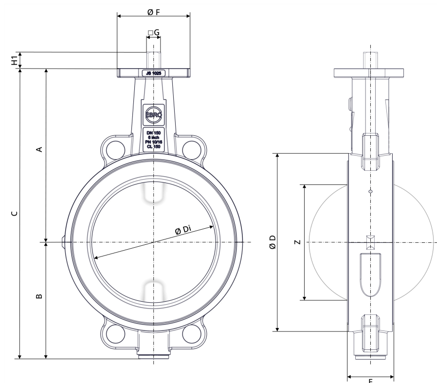
Figur 3: Hovedmål T211-A
