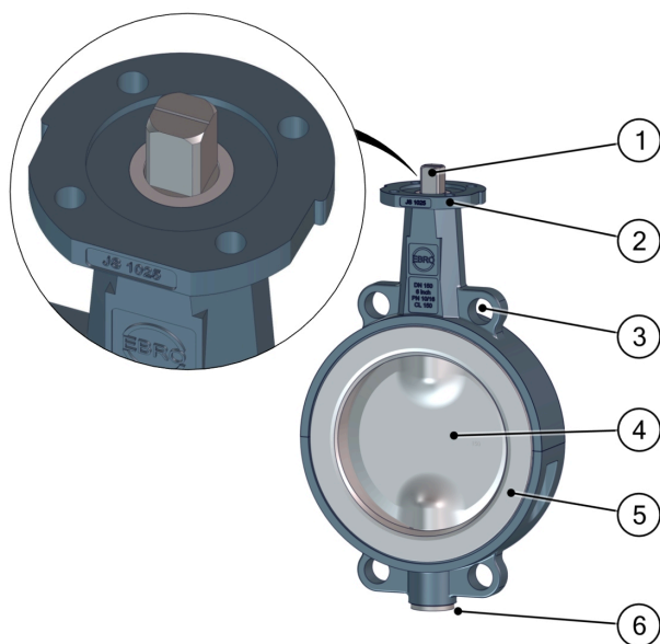
Figur 2: Benennung der Komponenten
