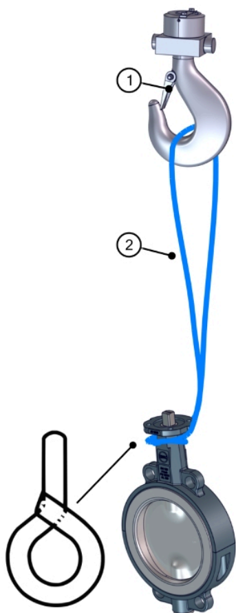
Figur 6: Zwischenflanschklappe kranen
