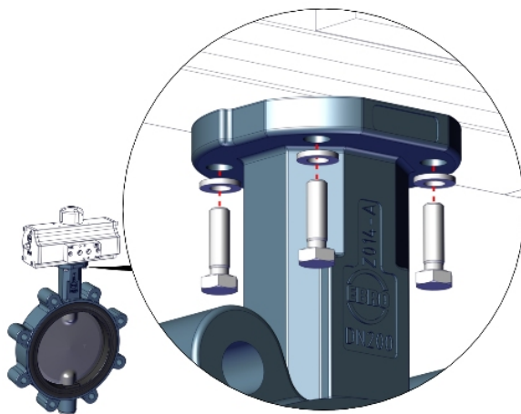
Figur 7: Princip monter komponenterne
