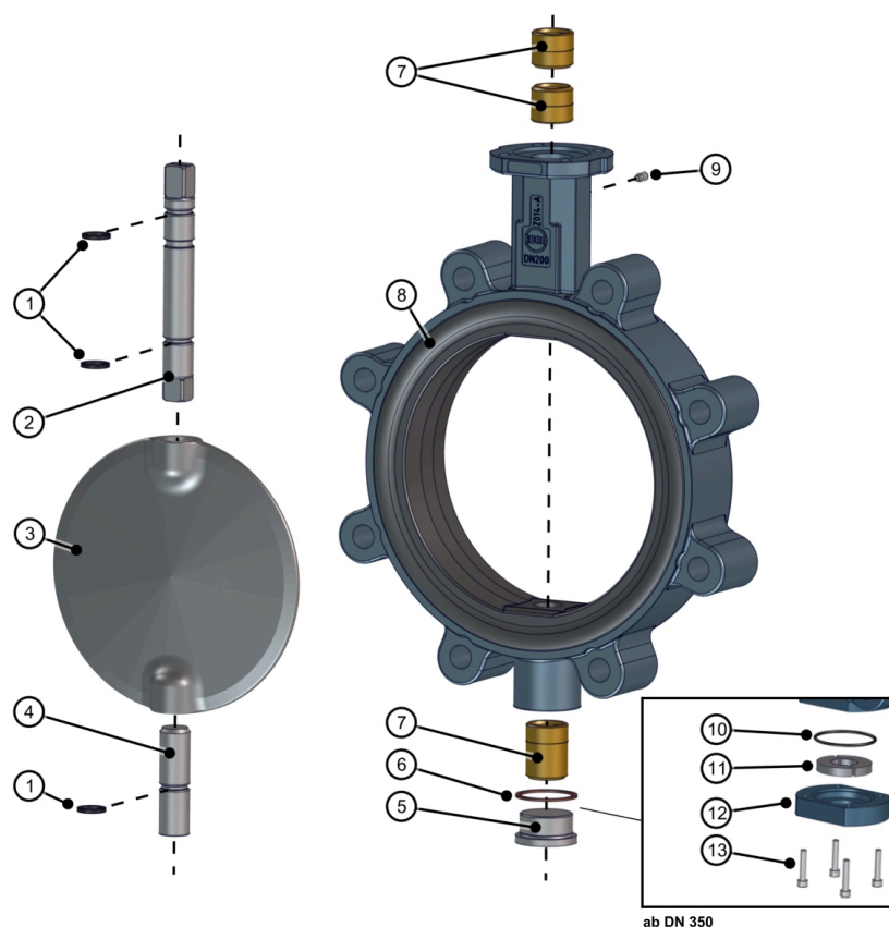
Figur 15: Stykliste Z014-B
