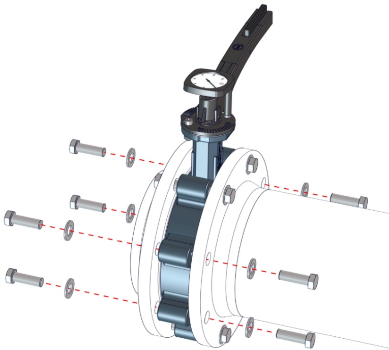
Figur 9: Skru sideflangeklappen fast
