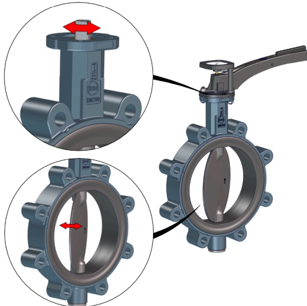
Figur 4: Bevægelige dele
