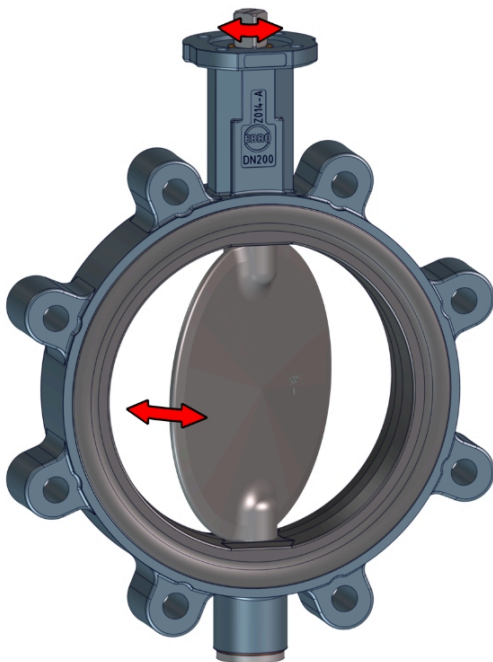
Figur 4: Bevægelige dele
