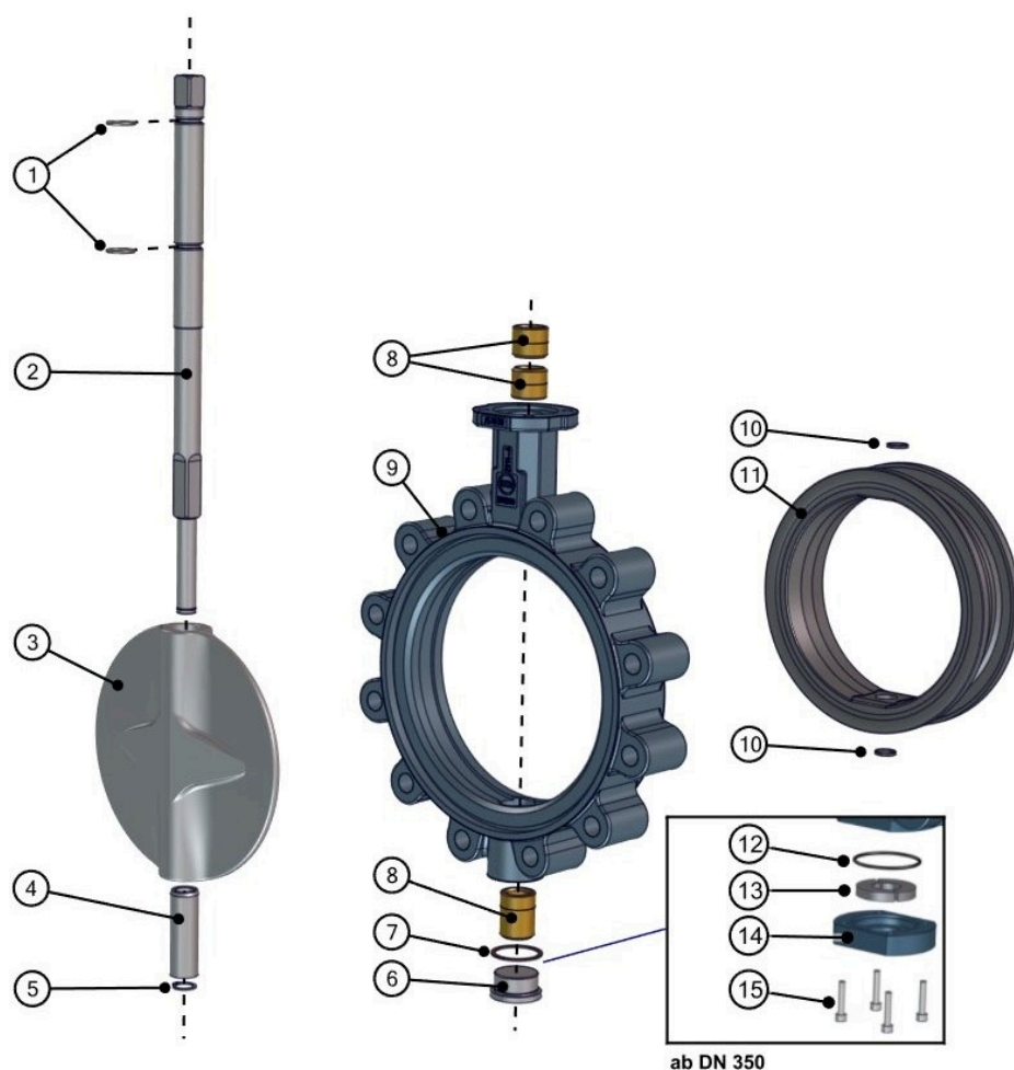
Figur 16: Stykliste Z014-A TS-aksel
