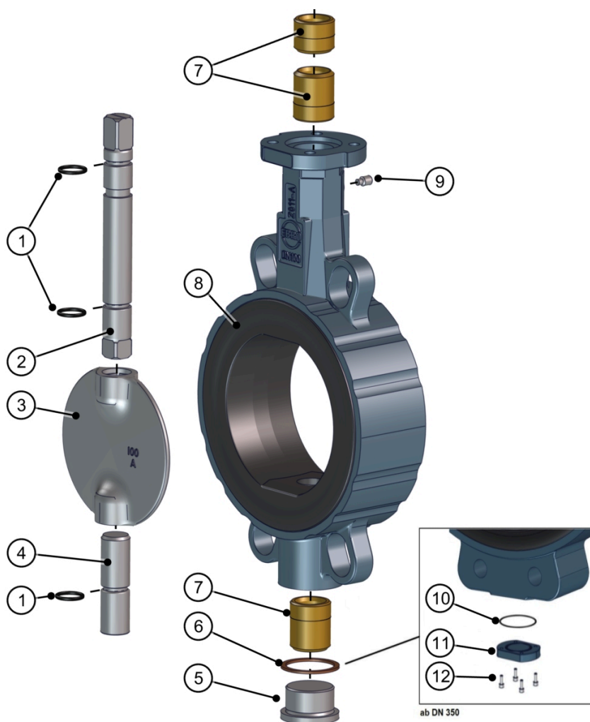
Figur 15: Stykliste Z011-B delt aksel
