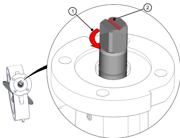
Figur 14: Betjeningsretning
