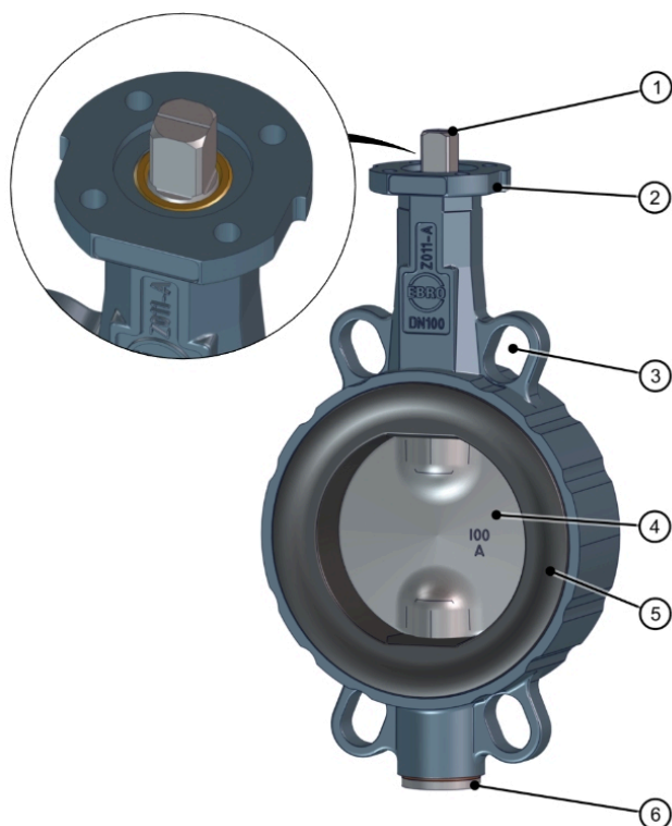
Figur 2: Komponenter
