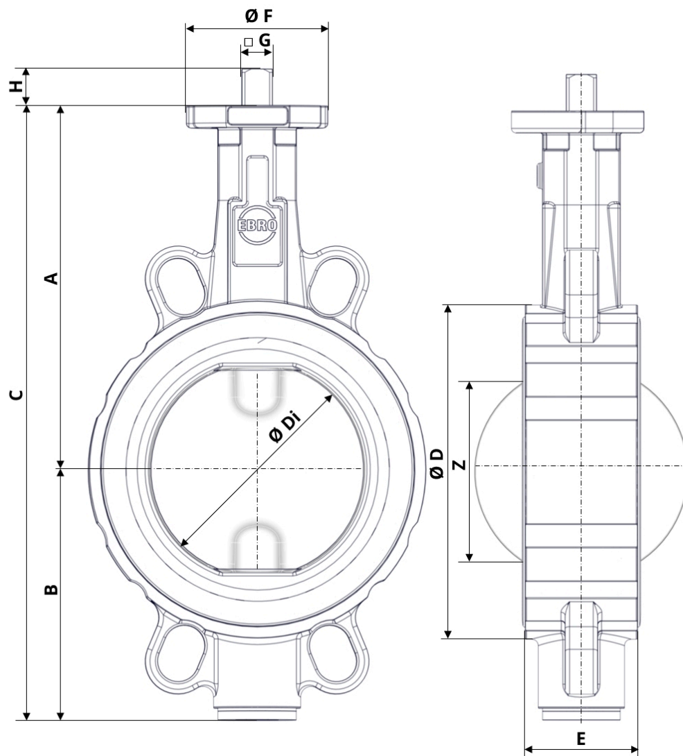
Figur 3: Hovedmål Z011-B
