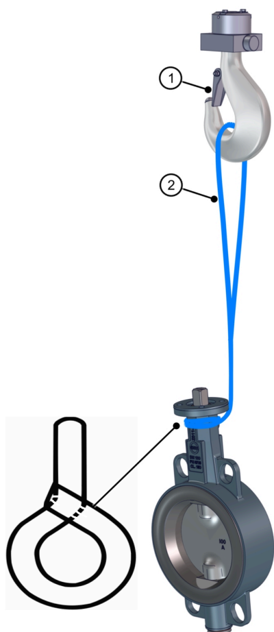
Figur 6: Løft mellemflangeklappen
