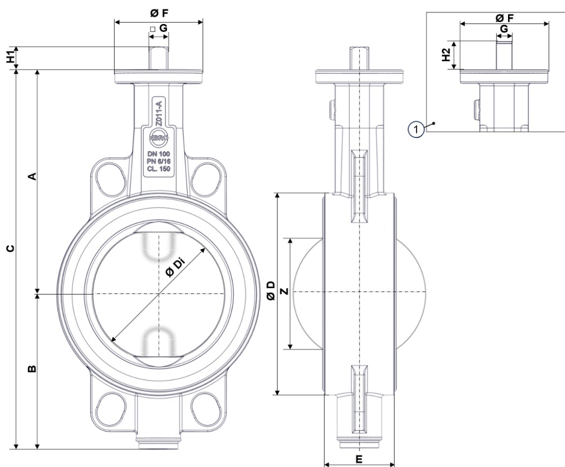
Figur 3: Hovedmål Z011-AS
