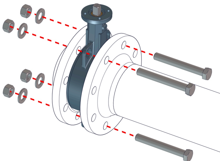
Figur 8: Placer mellemlangeklap
