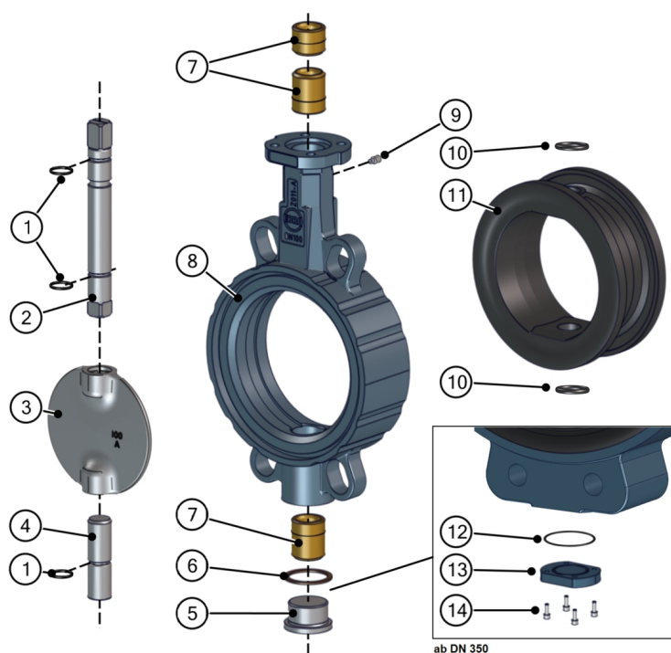
Figur 15: Stykliste Z011-A delt aksel
