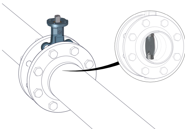
Figur 13: Skyl rør
