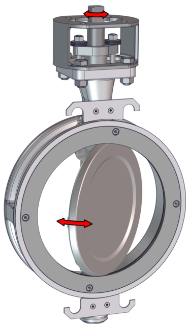
Obr. 4: Pohyblivé díly
