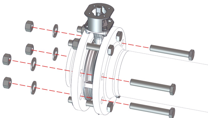
Obr. 9: Přišroubovat klapku vložené příruby
