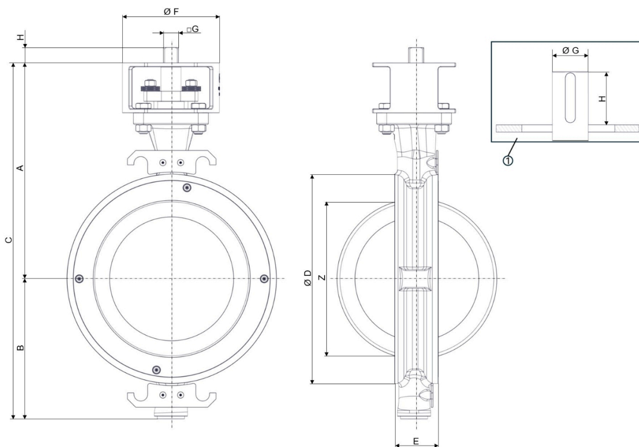
Obr. 3: Hlavní rozměry HP111
