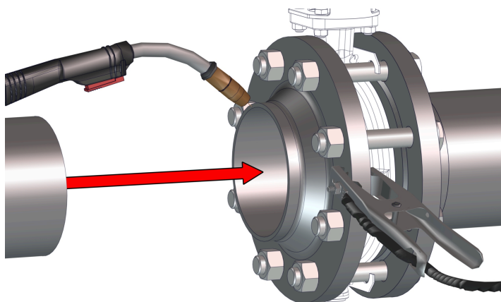
Obr. 10: Svaření potrubí s přírubou
