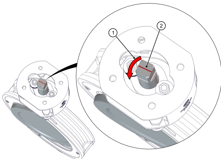
Obr. 14: Směr ovládání
