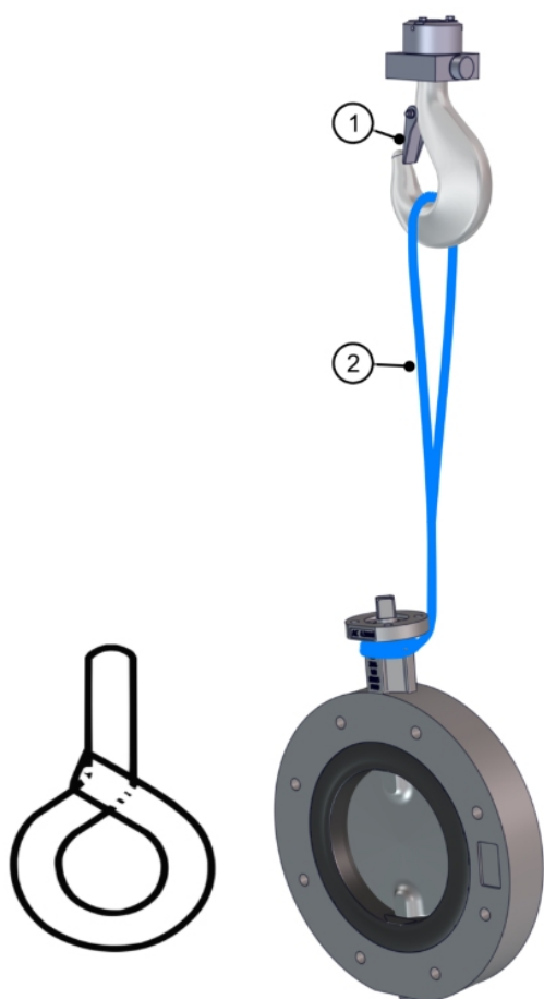
Obr. 6: Přepravte klapku plné příruby jeřábem
