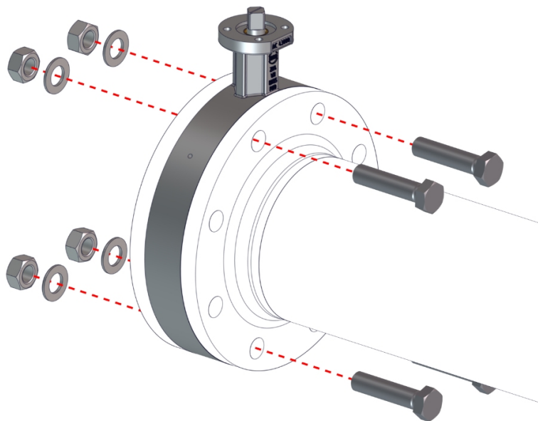
Obr. 8: Polohování klapky plné příruby
