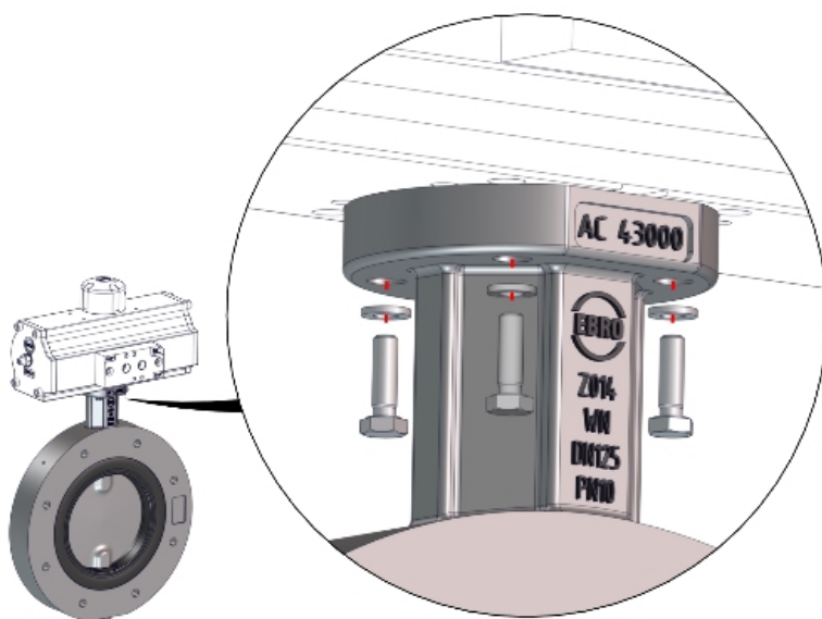
Obr. 7: Princip montáže komponent
