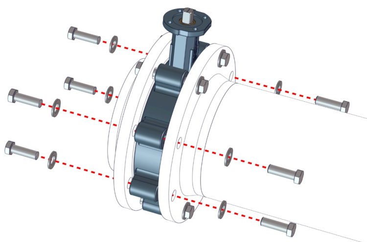
Obr. 9: Přišroubování klapky příruby
